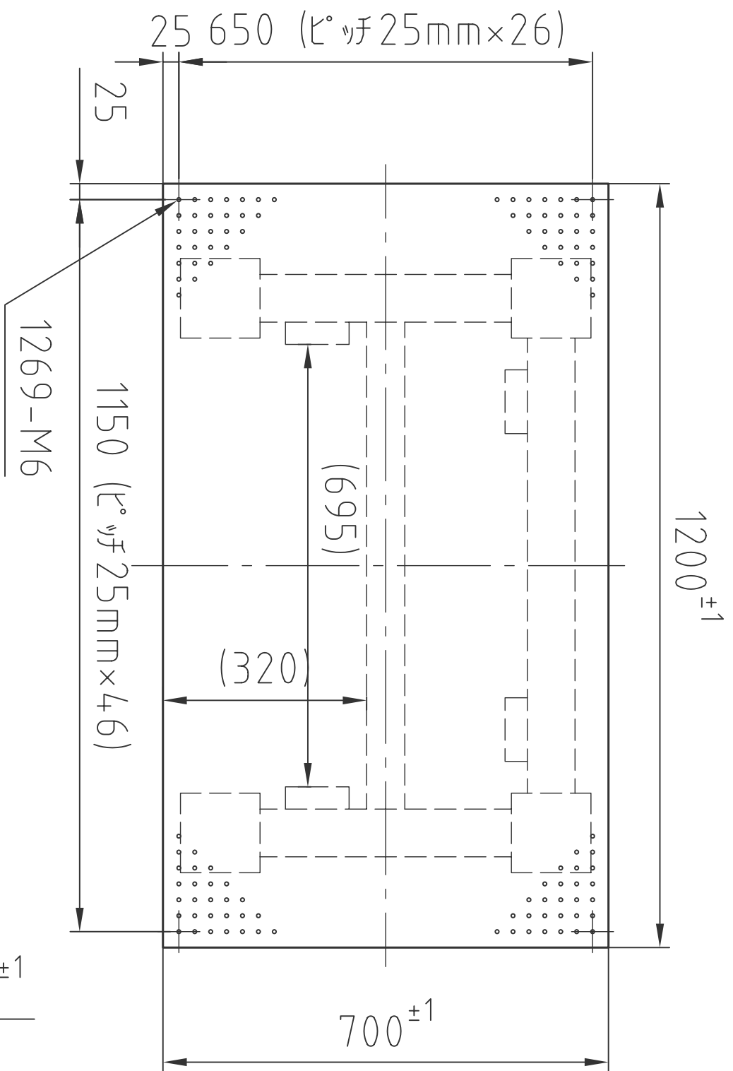
(平面図)
