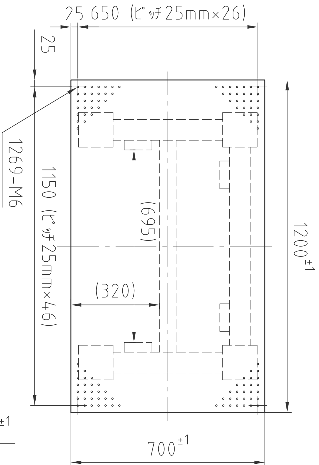
(平面図)
