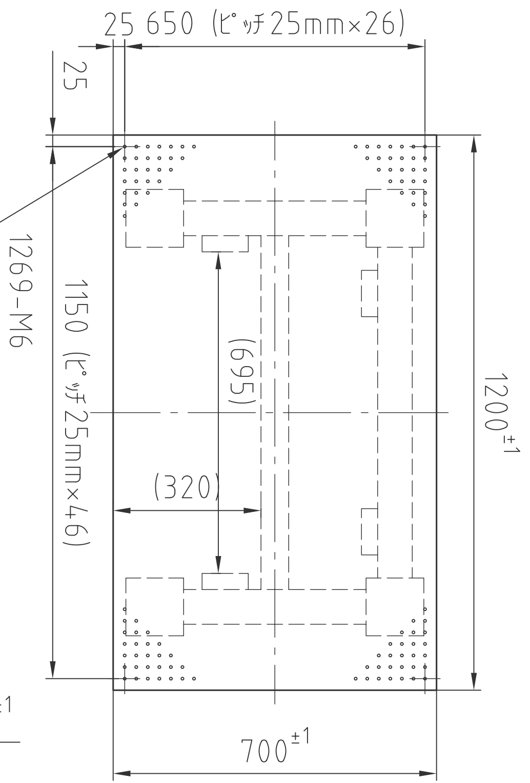
(平面図)
