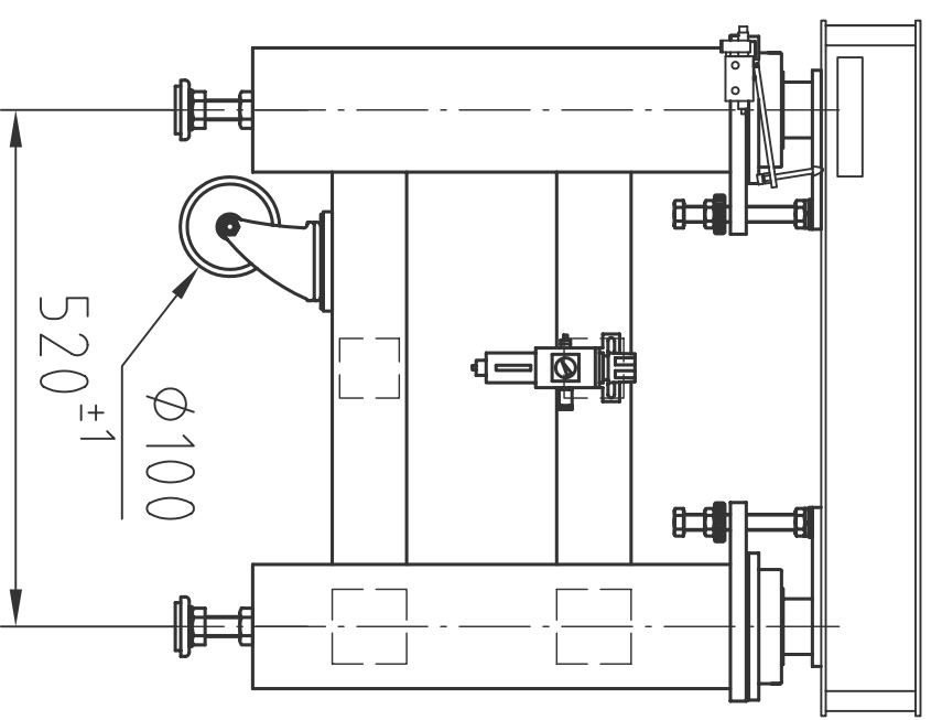
(右側面図)
