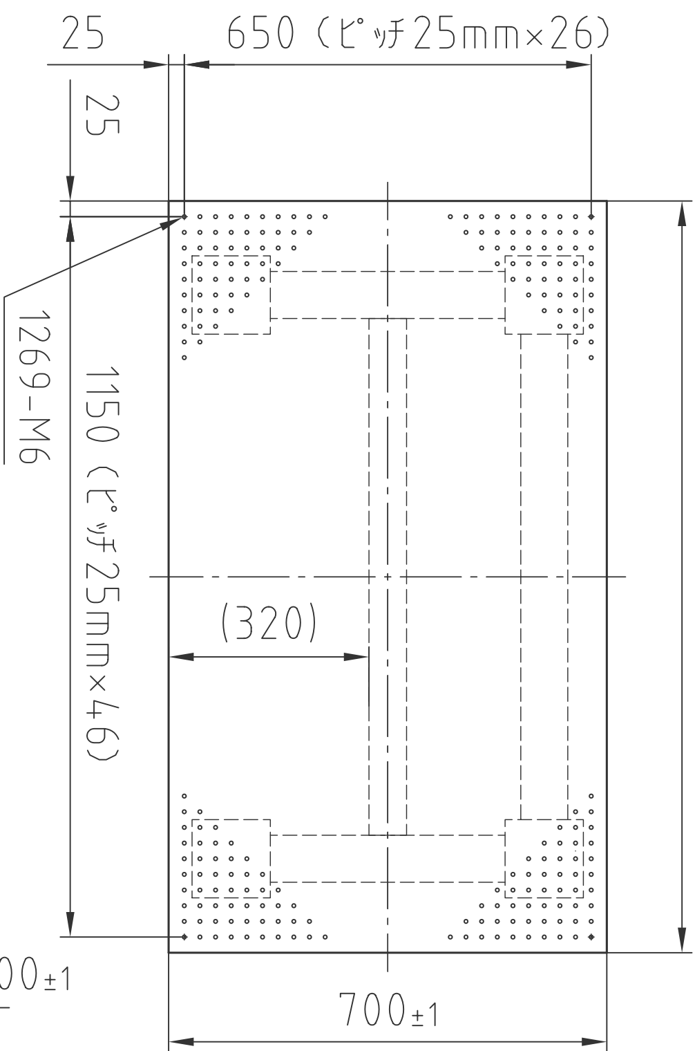
(平面図)
