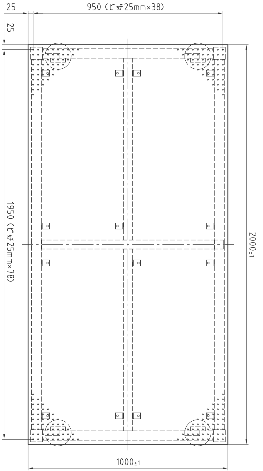
(正面図)
