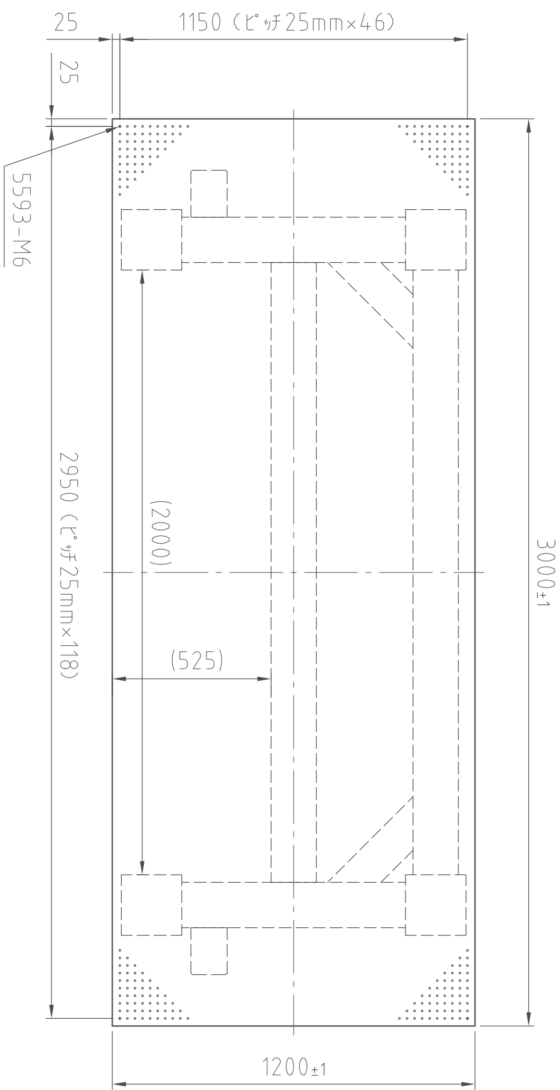
(平面図)
