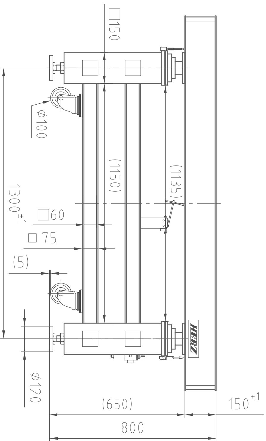
(正面図)
