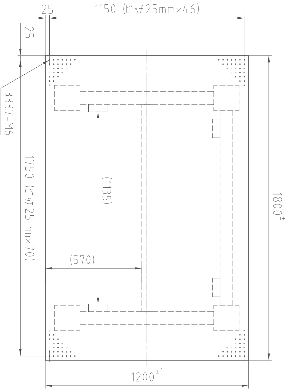
(平面図)
