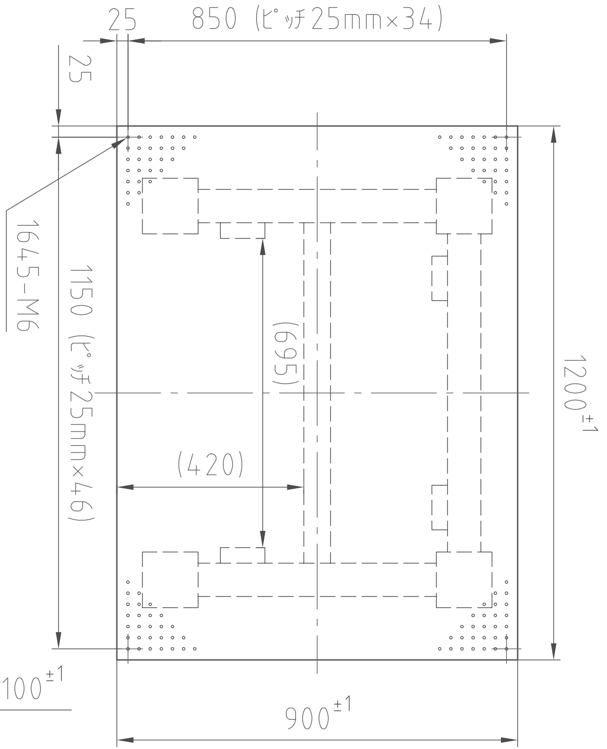
(平面図)
