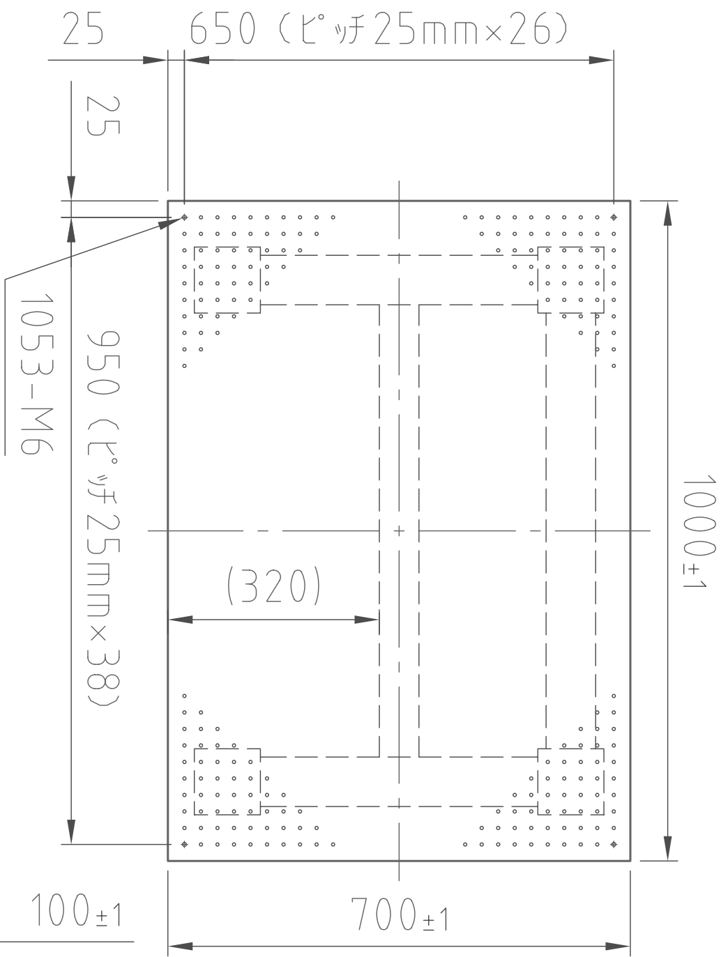
(平面図)
