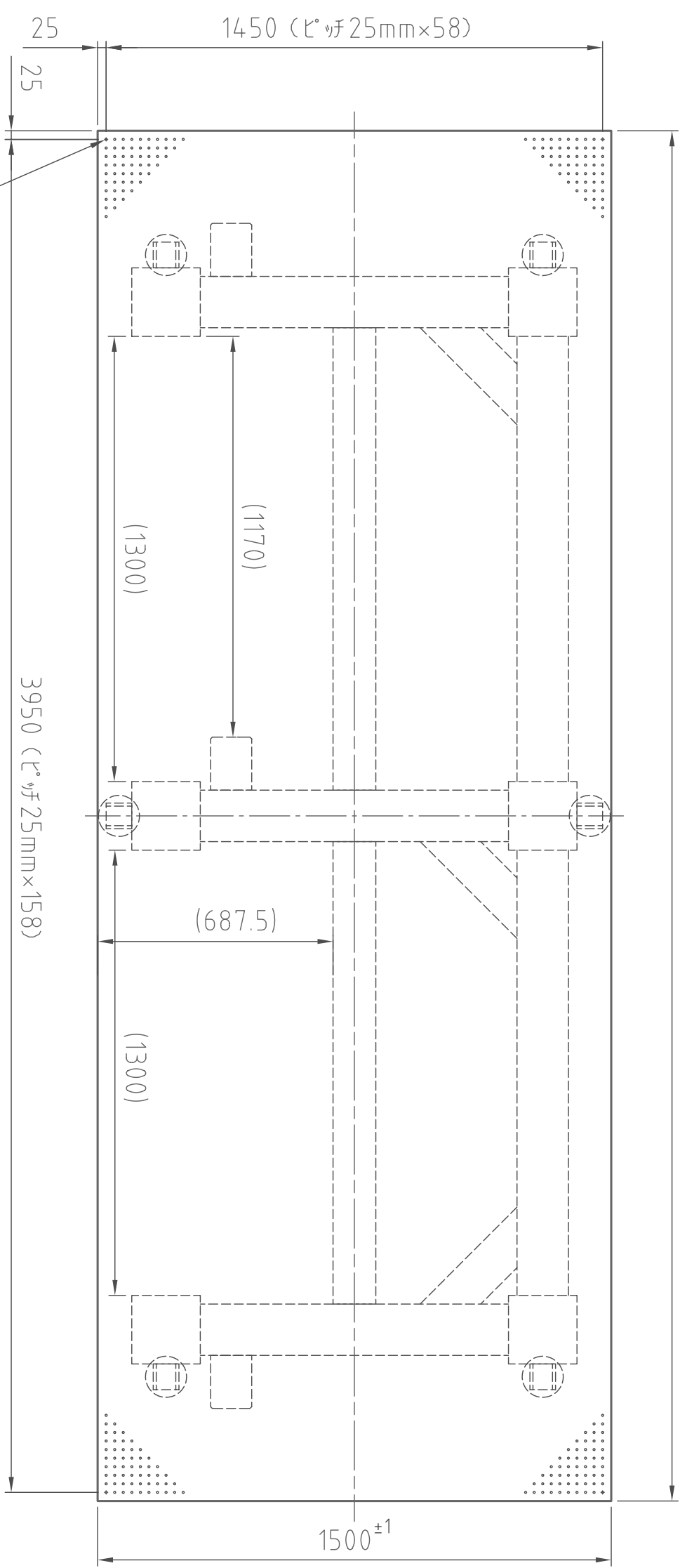
(平面图)
