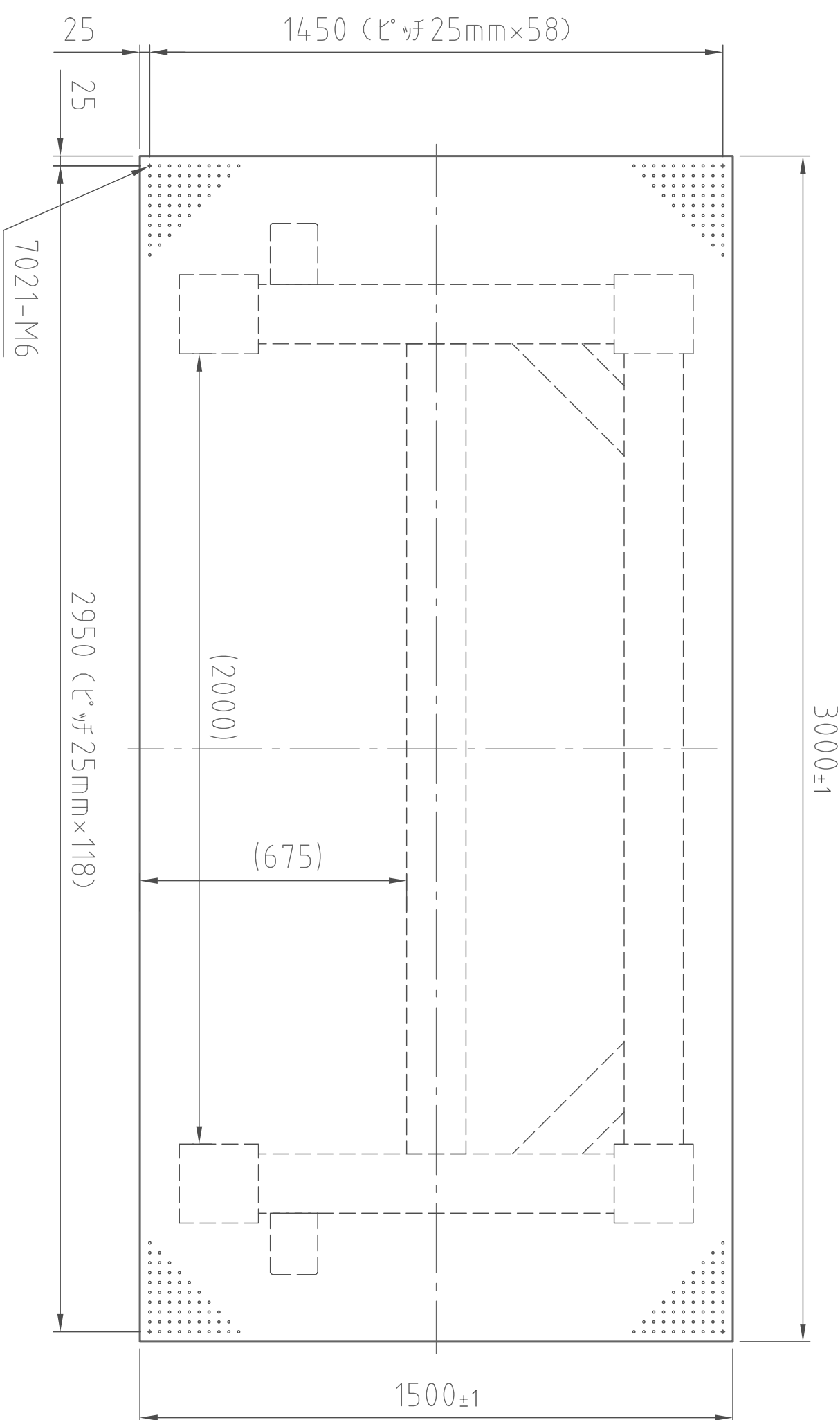
(平面図)
