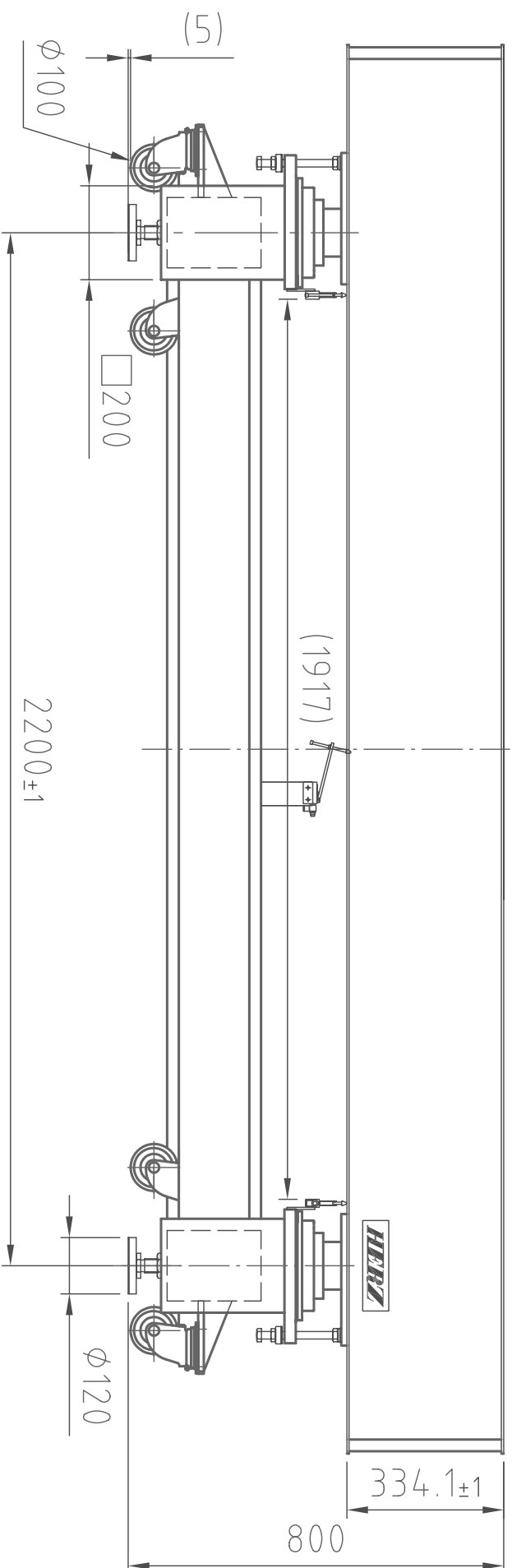
(正面図)
