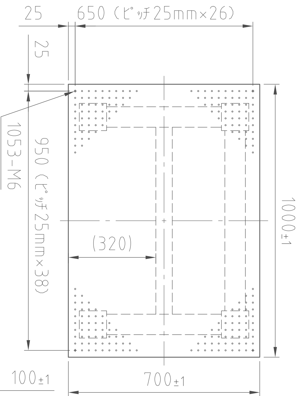
(平面図)
