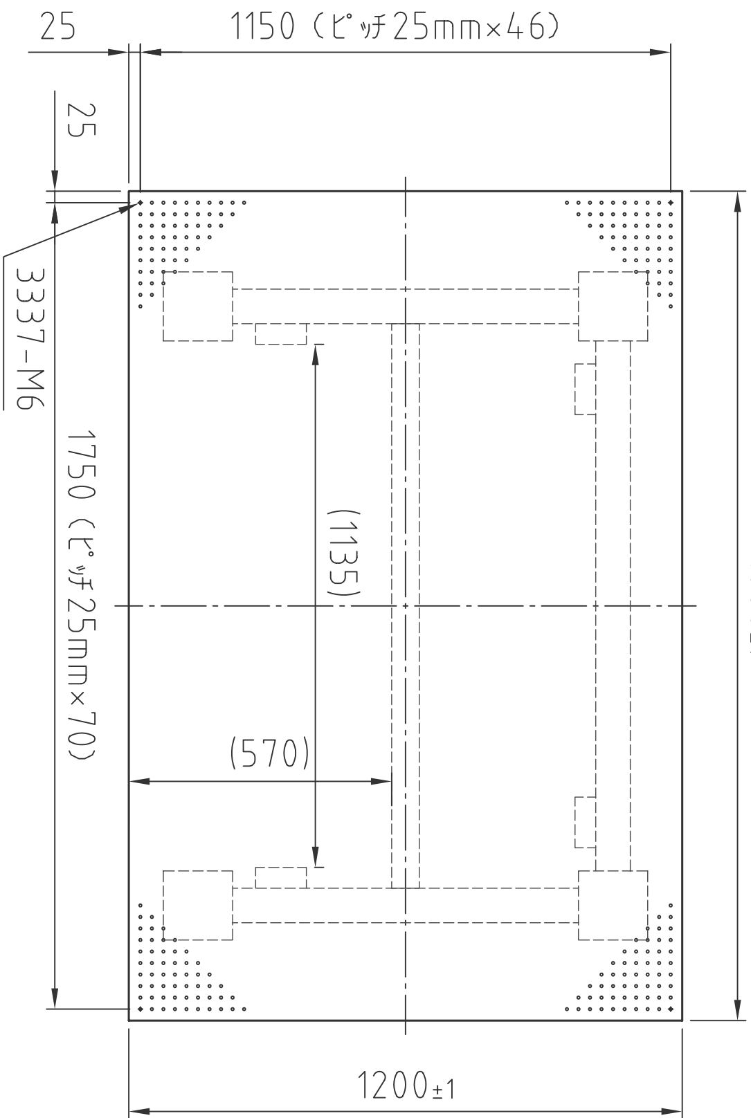
(平面図)
