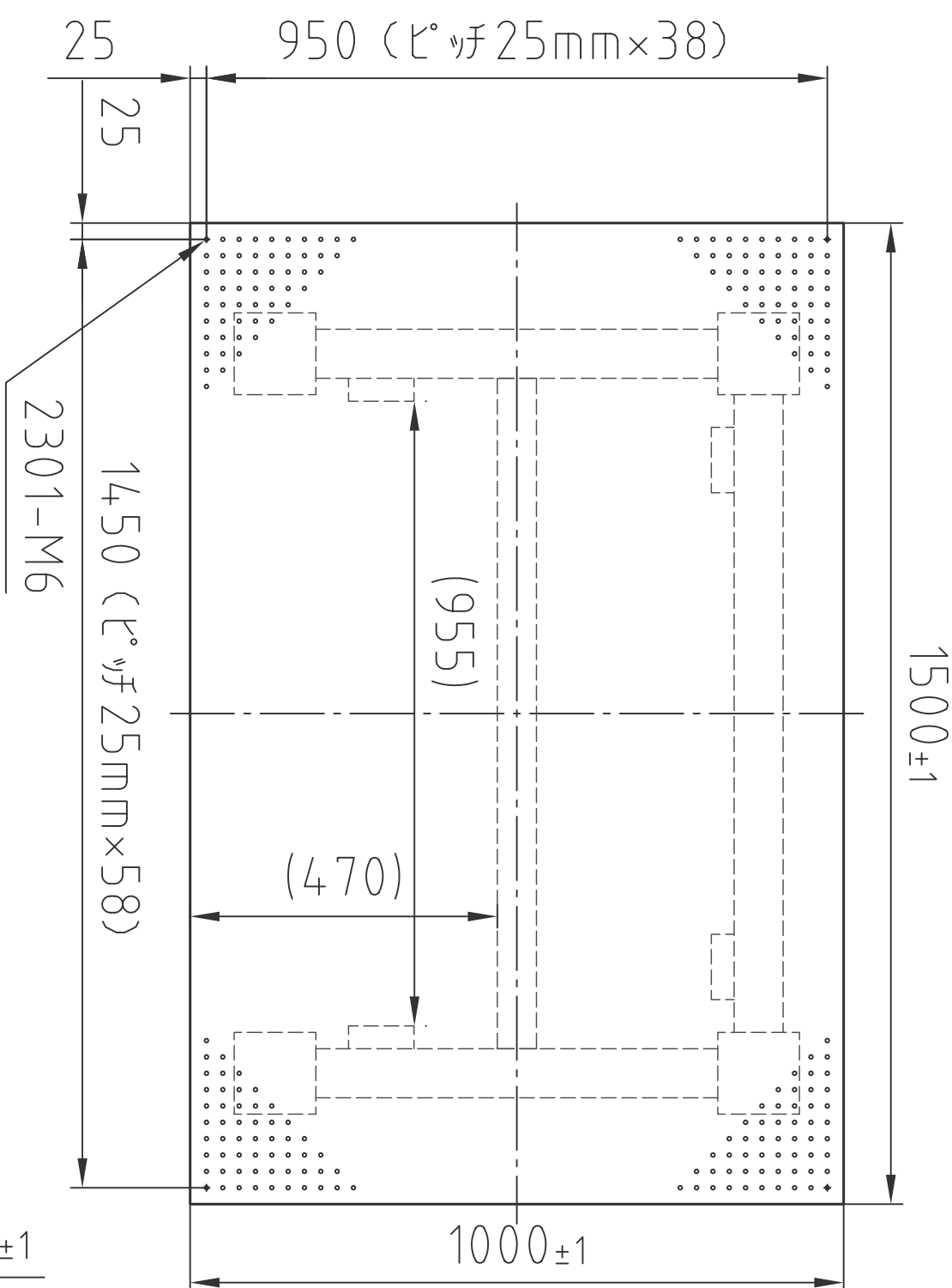
(平面図)
