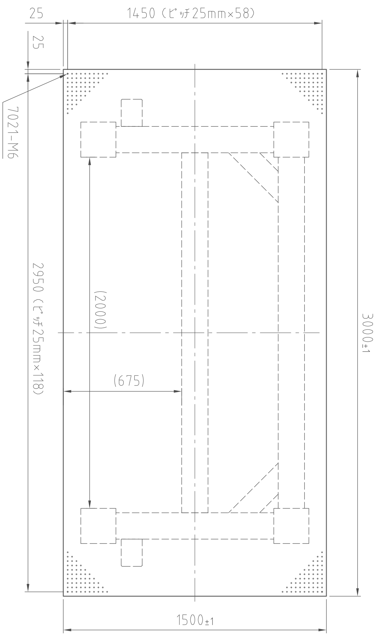
(平面図)
