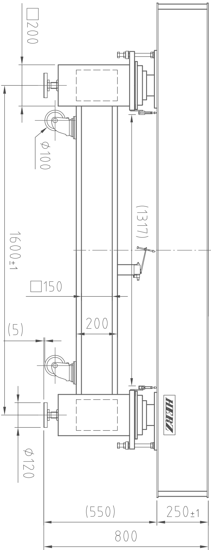
(正面図)
