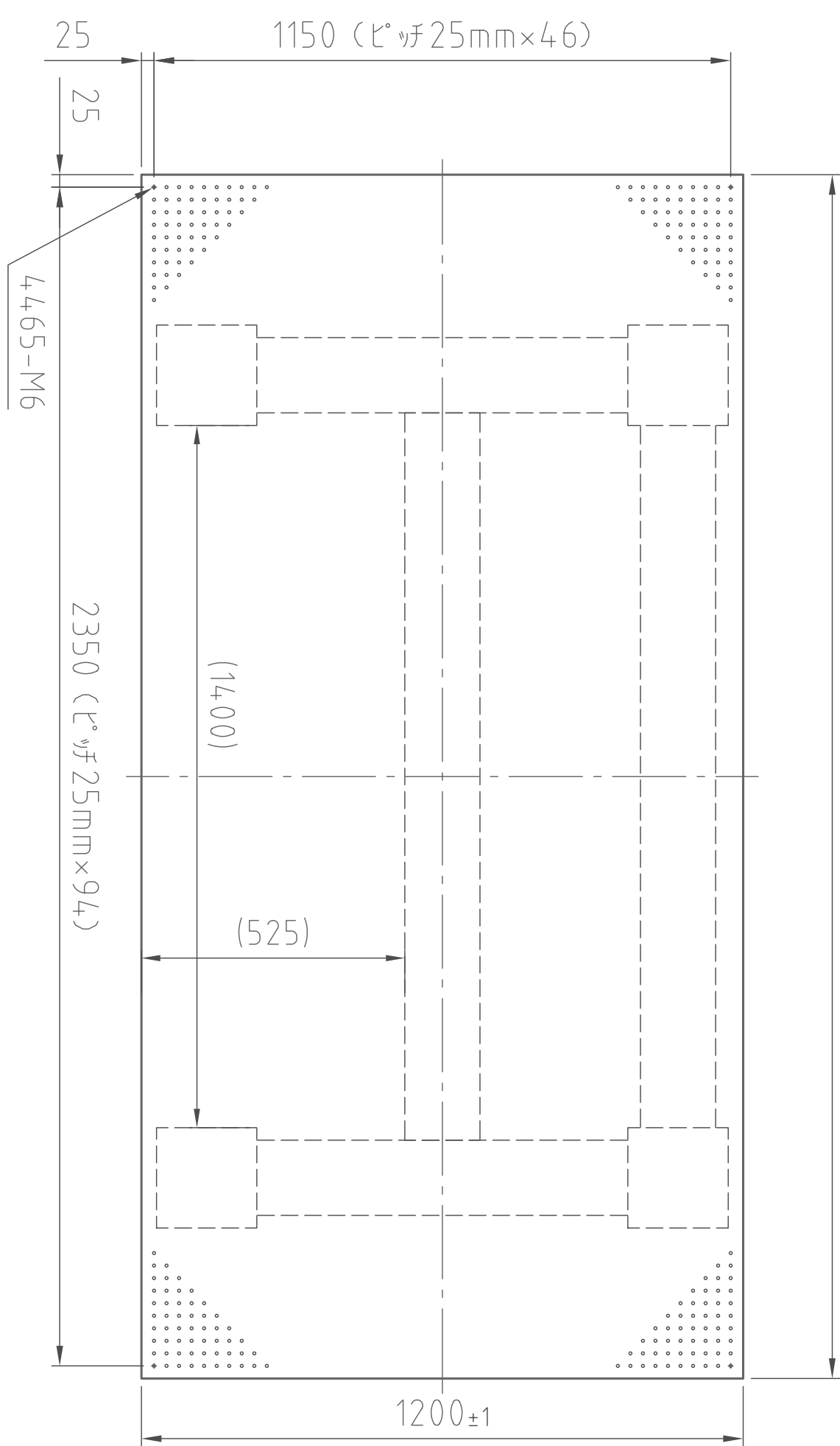
(平面図)
