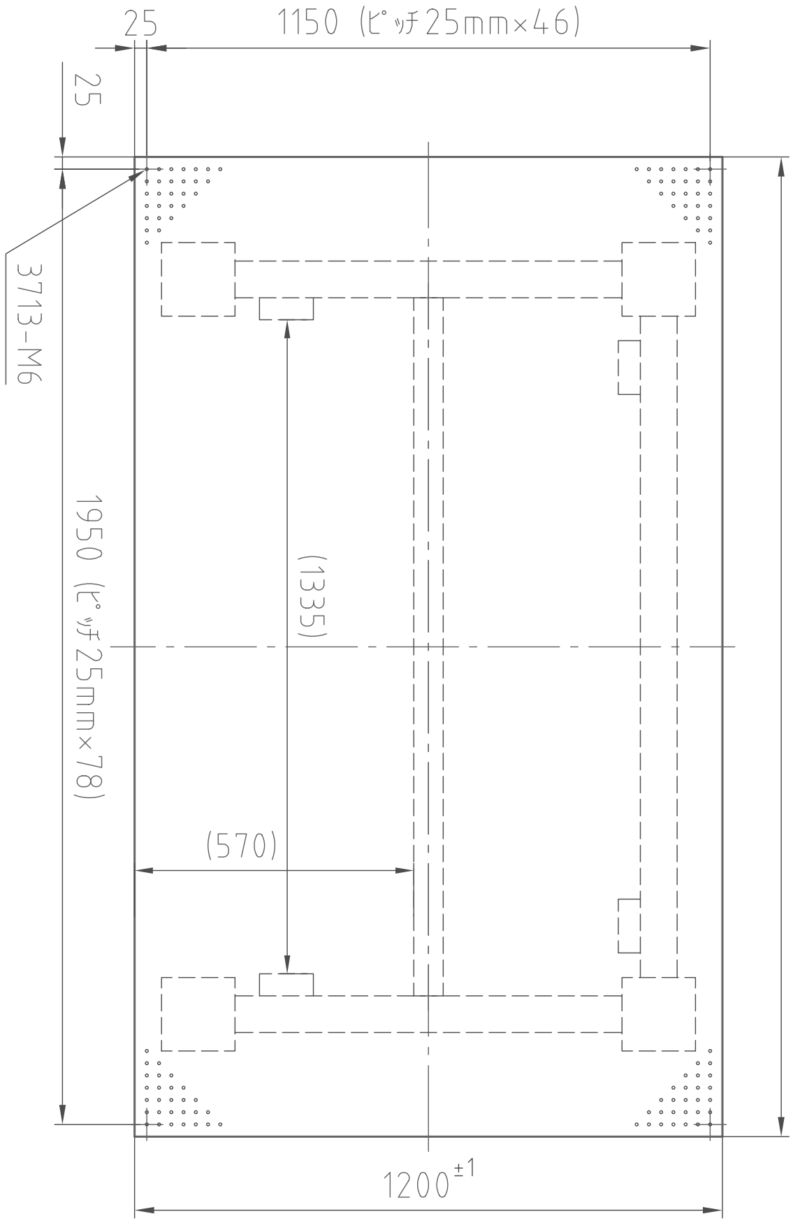
(平面図)
