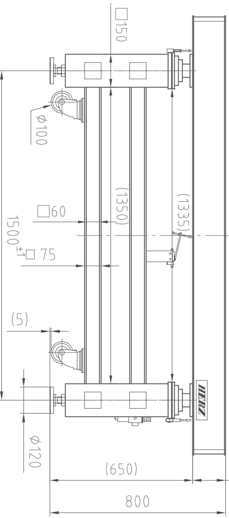
(正面図)
