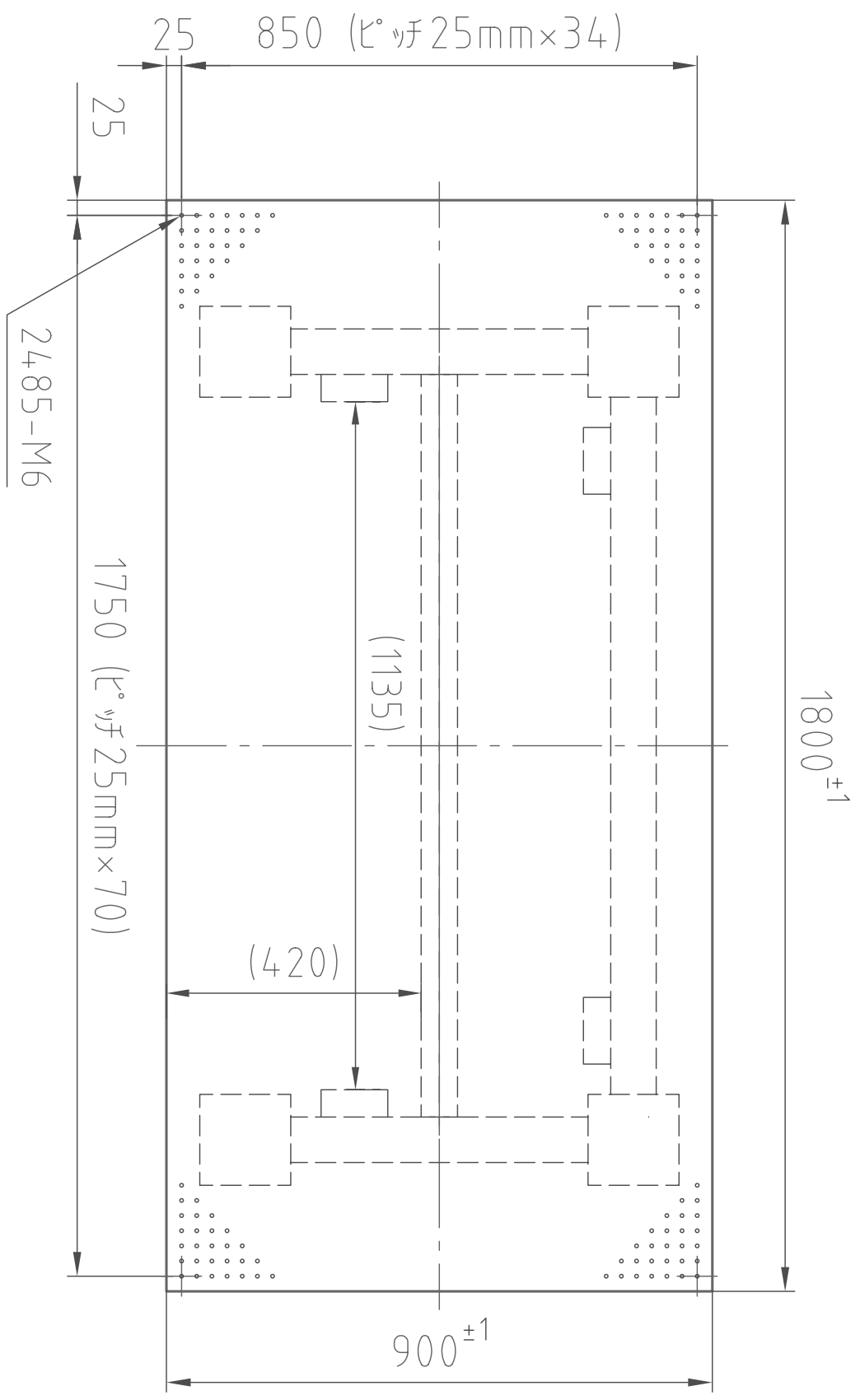
(平面図)
