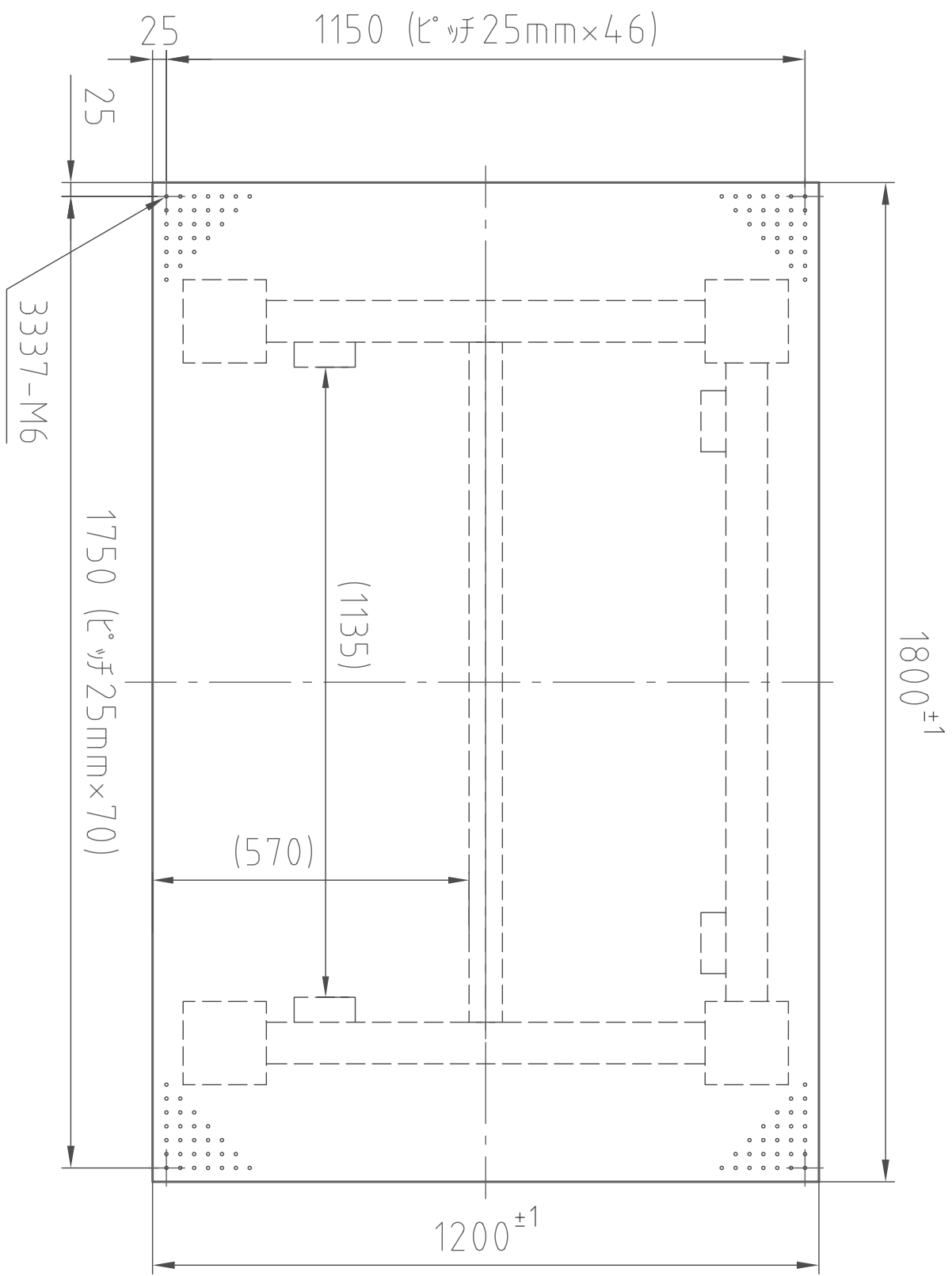
(平面図)
