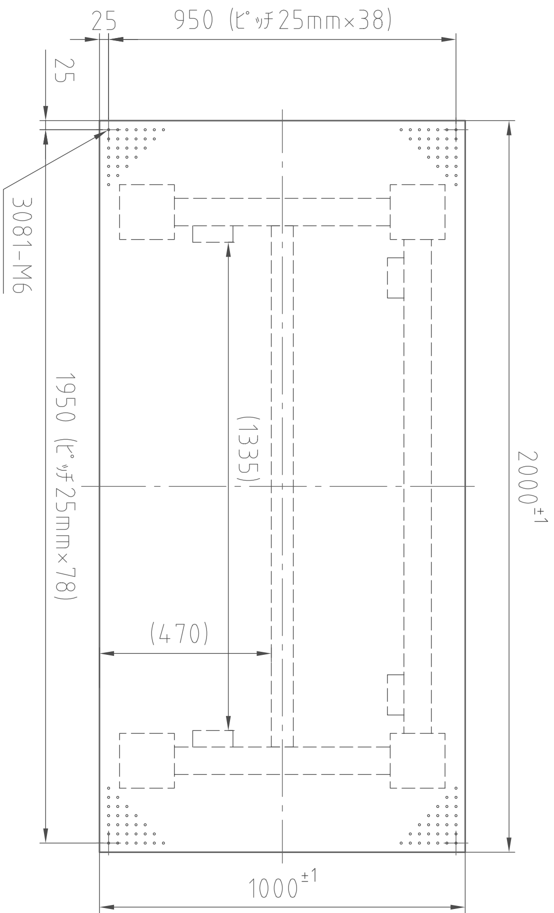
(平面図)
