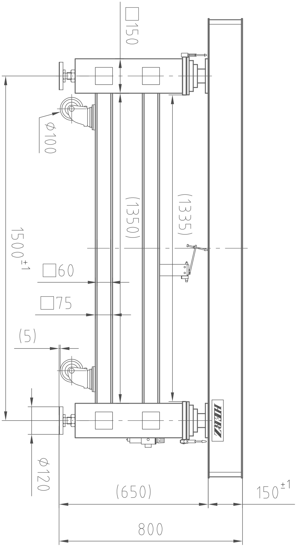
(正面図)
