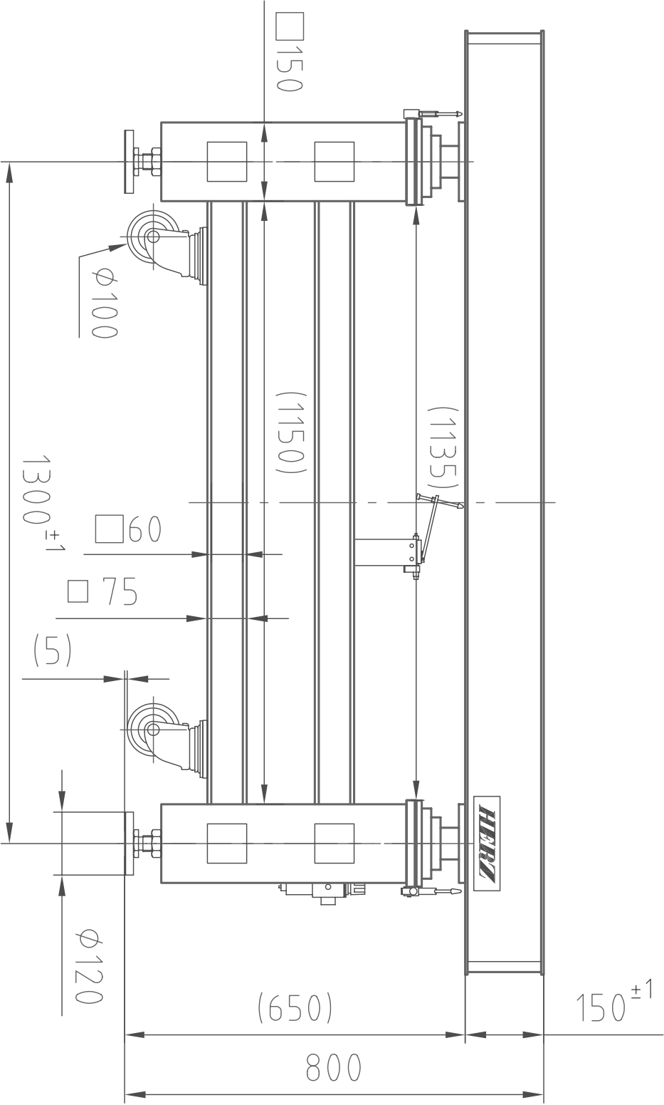
(正面図)
