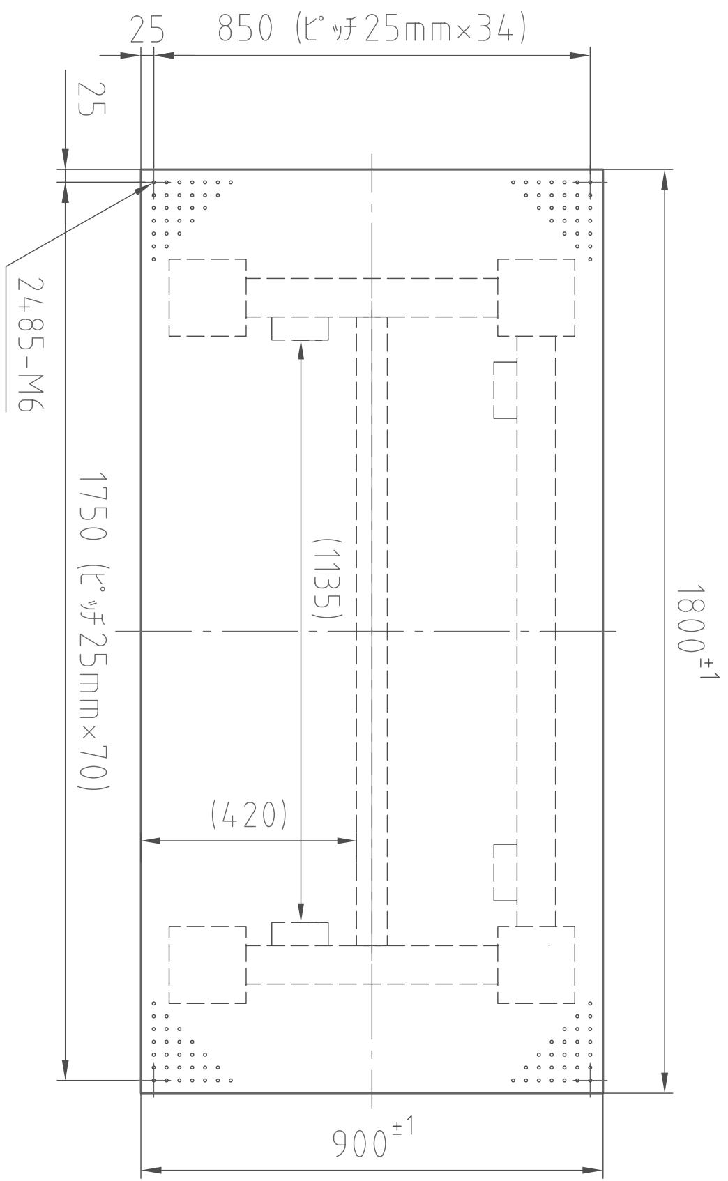
(平面図)
