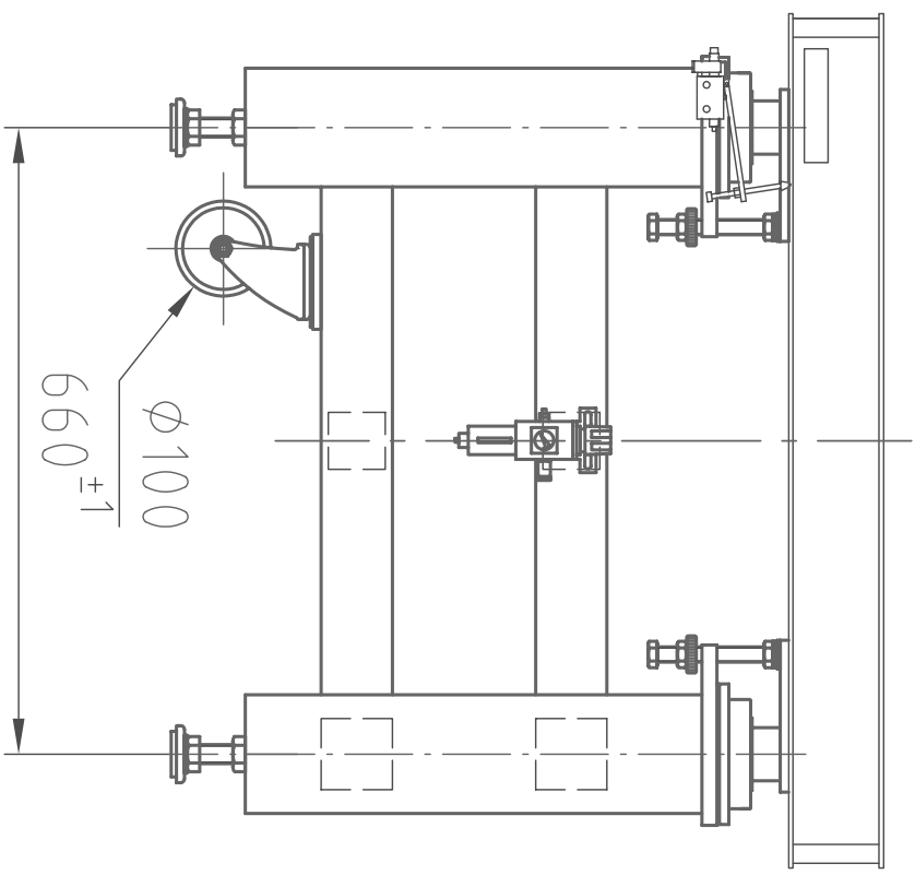
(右側面図)
