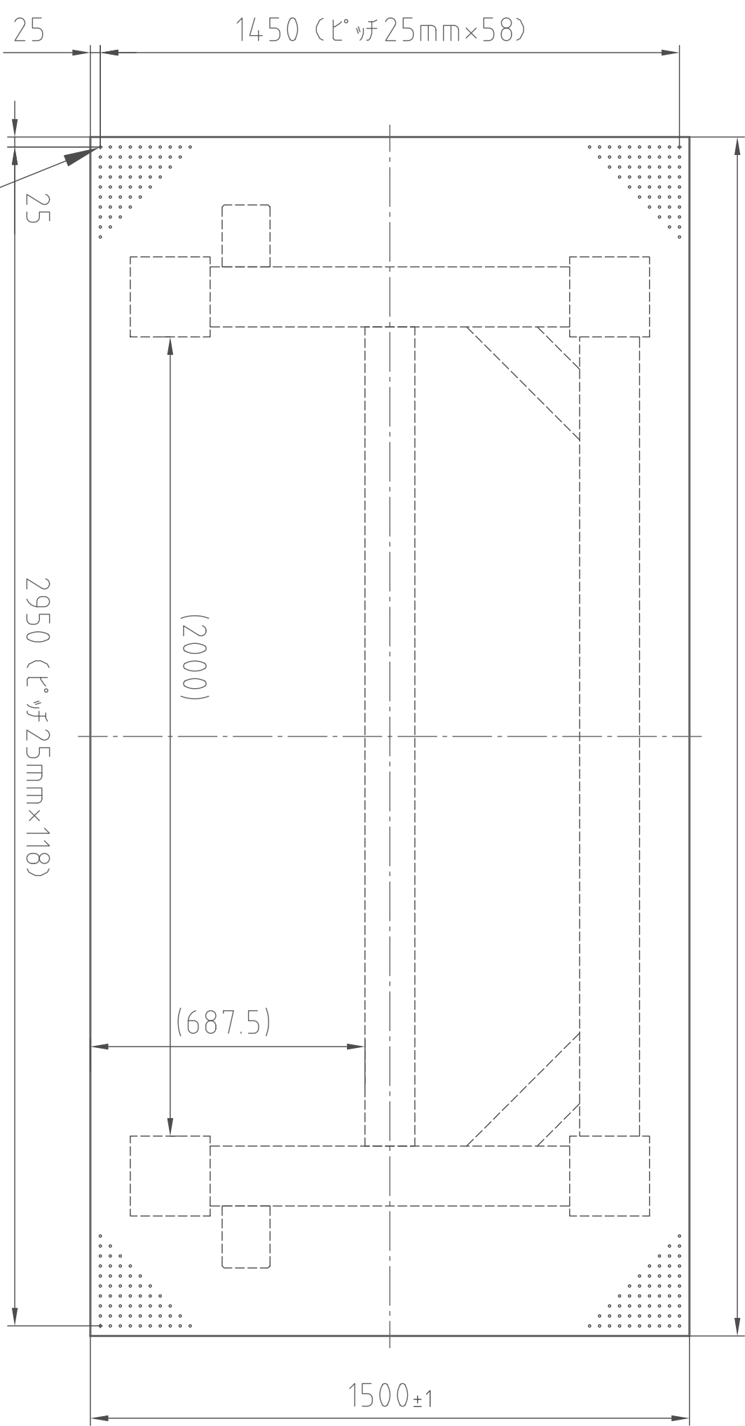
(平面図)
