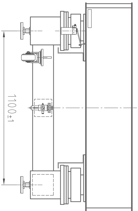
(右側面図)
