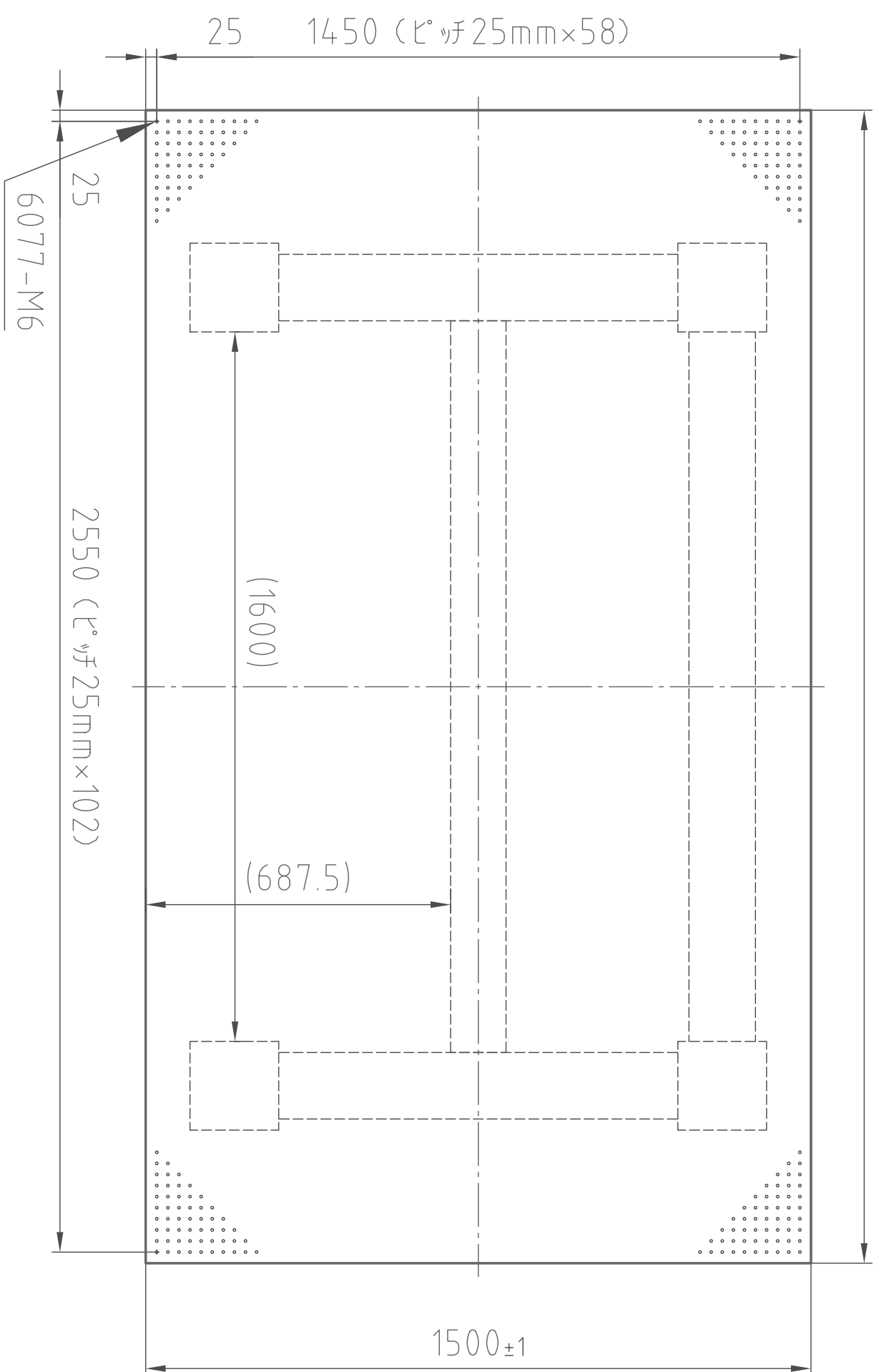
(平面図)
