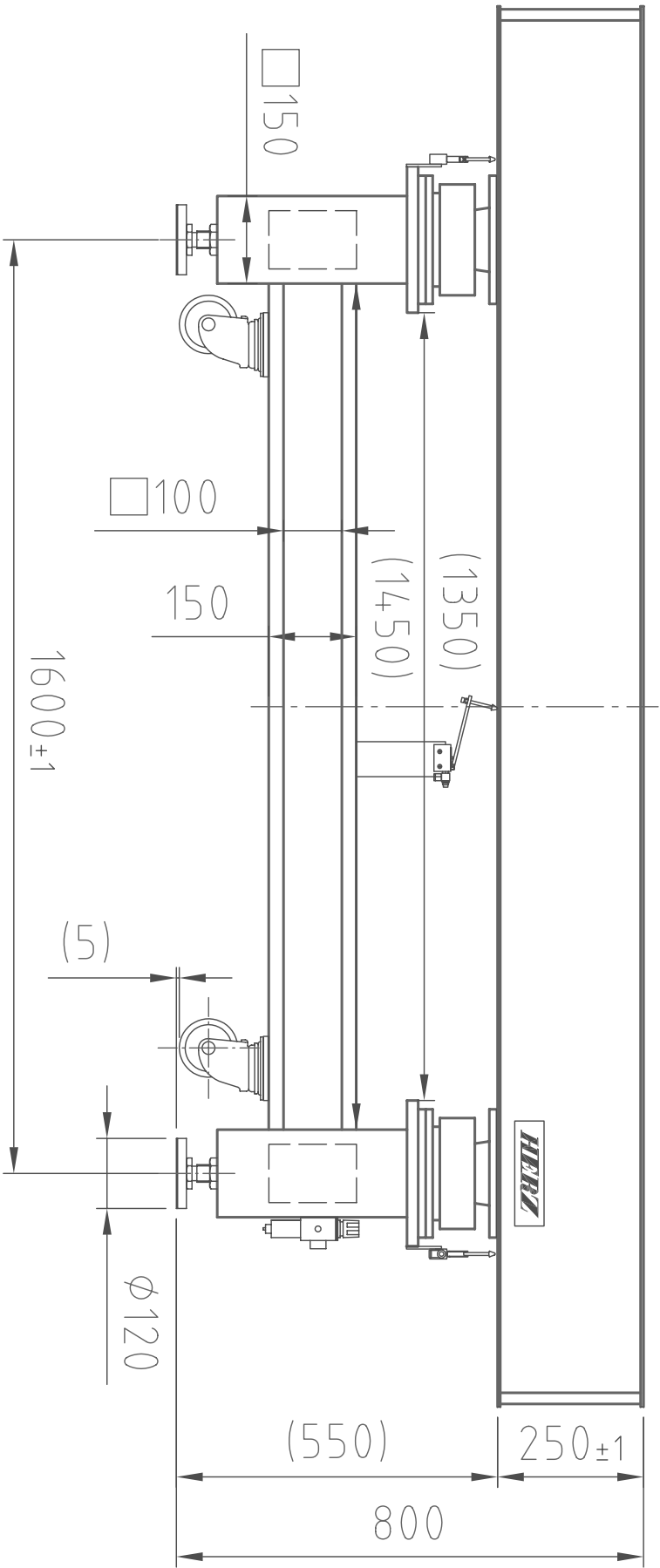
(正面図)
