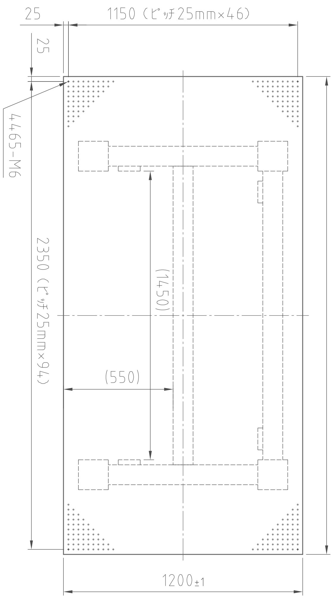
(平面図)
