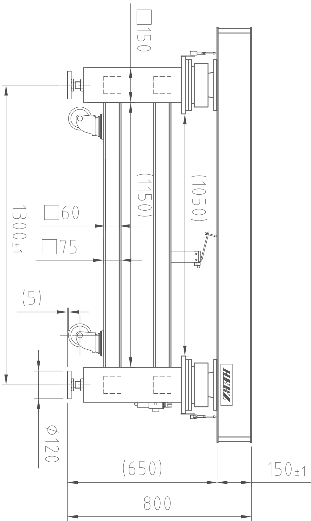
(正面図)
