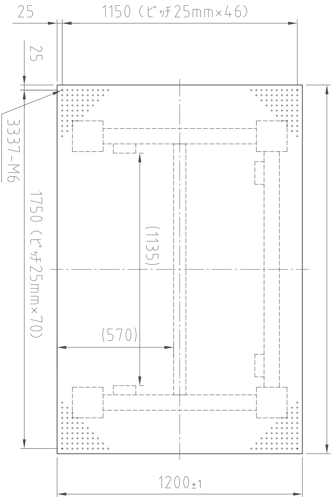
(平面図)
