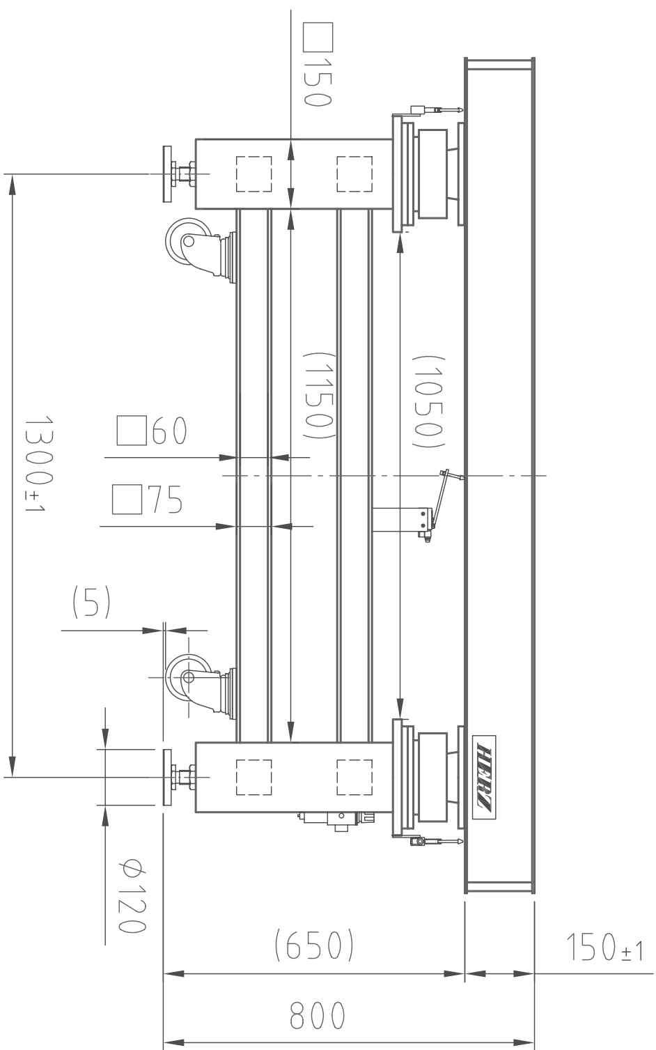
(正面図)
