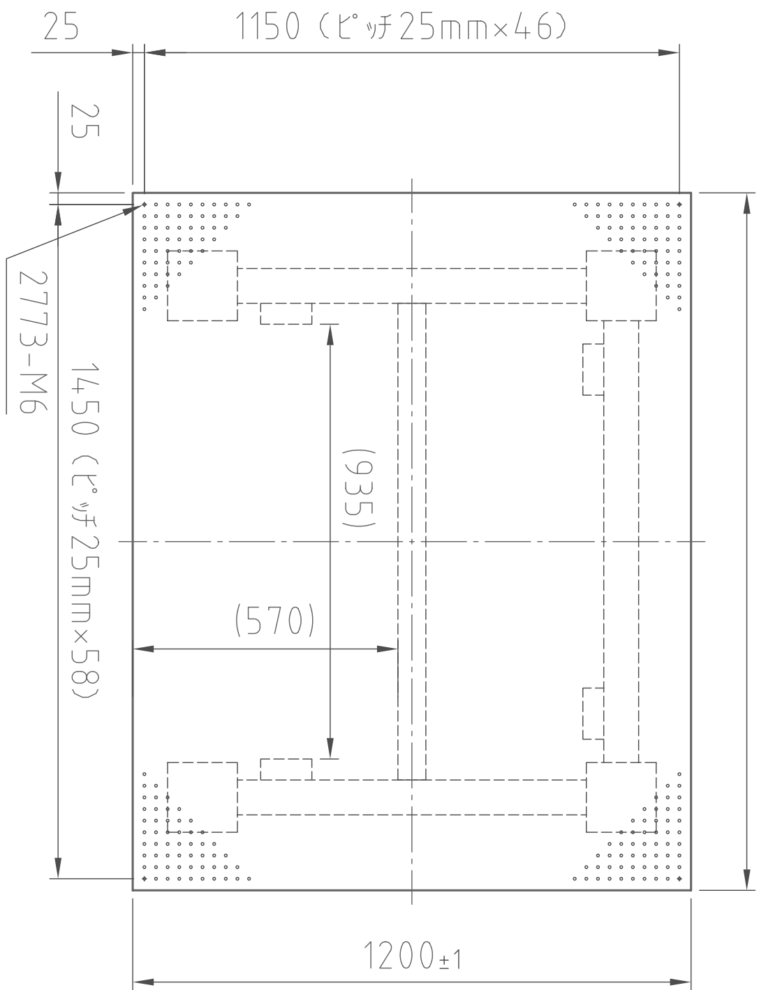
(平面図)
