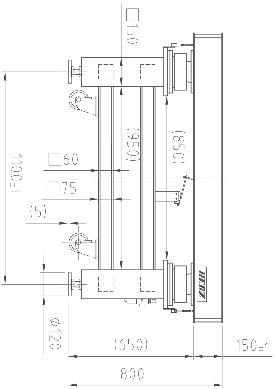
(正面図)
