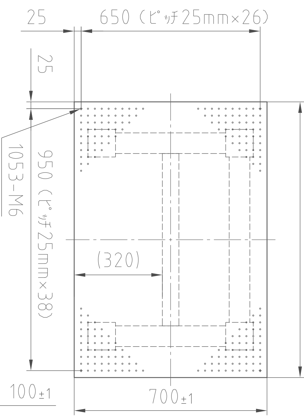
(平面図)
