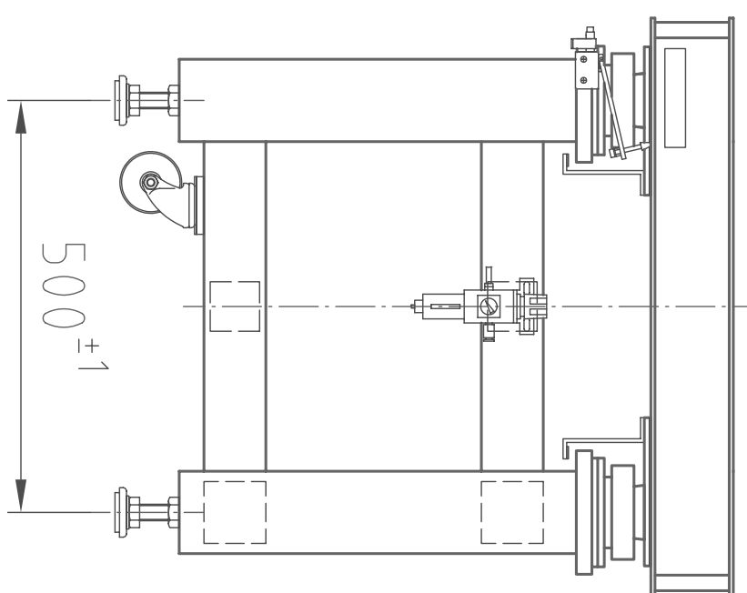
(右側面図)
