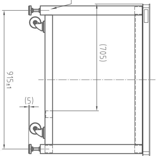
(右側面図)
