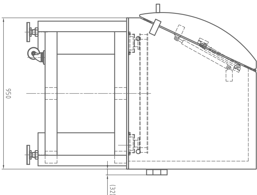
(右側面図)
