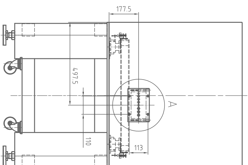
(背面図)
