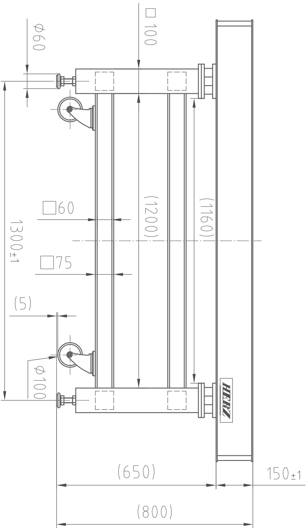
(正面図)
