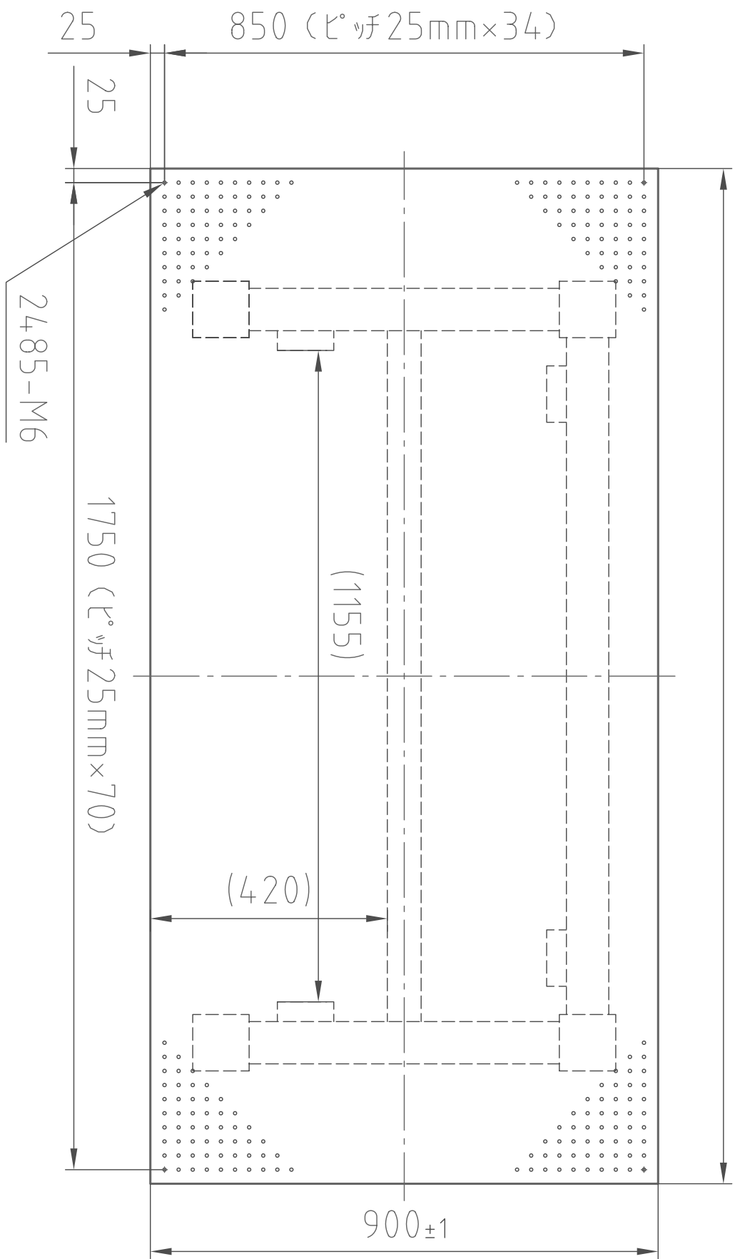
(平面図)
