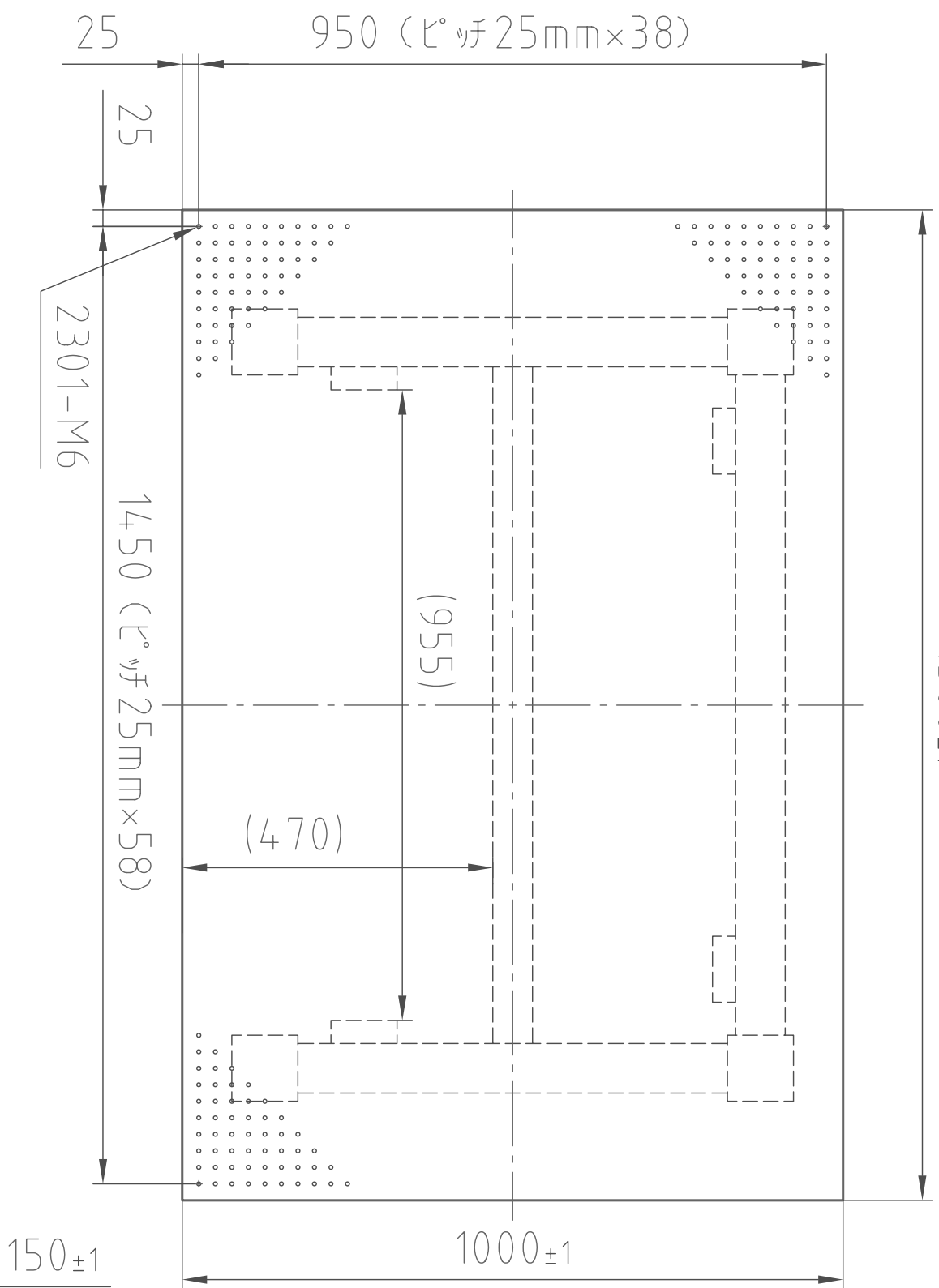
(平面図)
