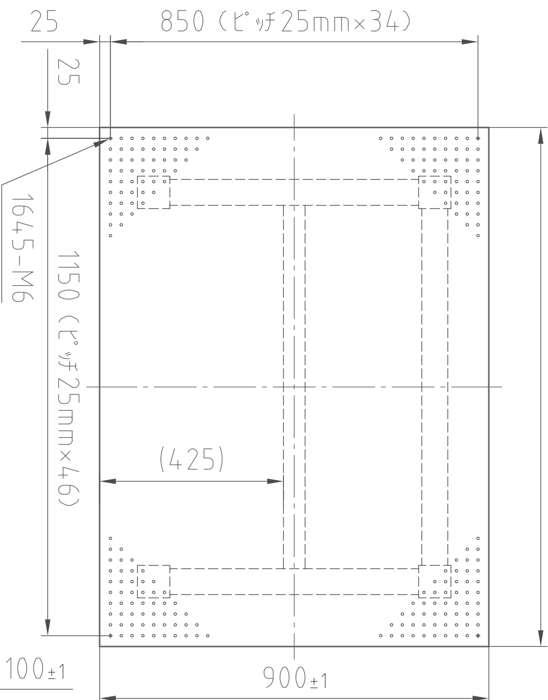
(平面図)
