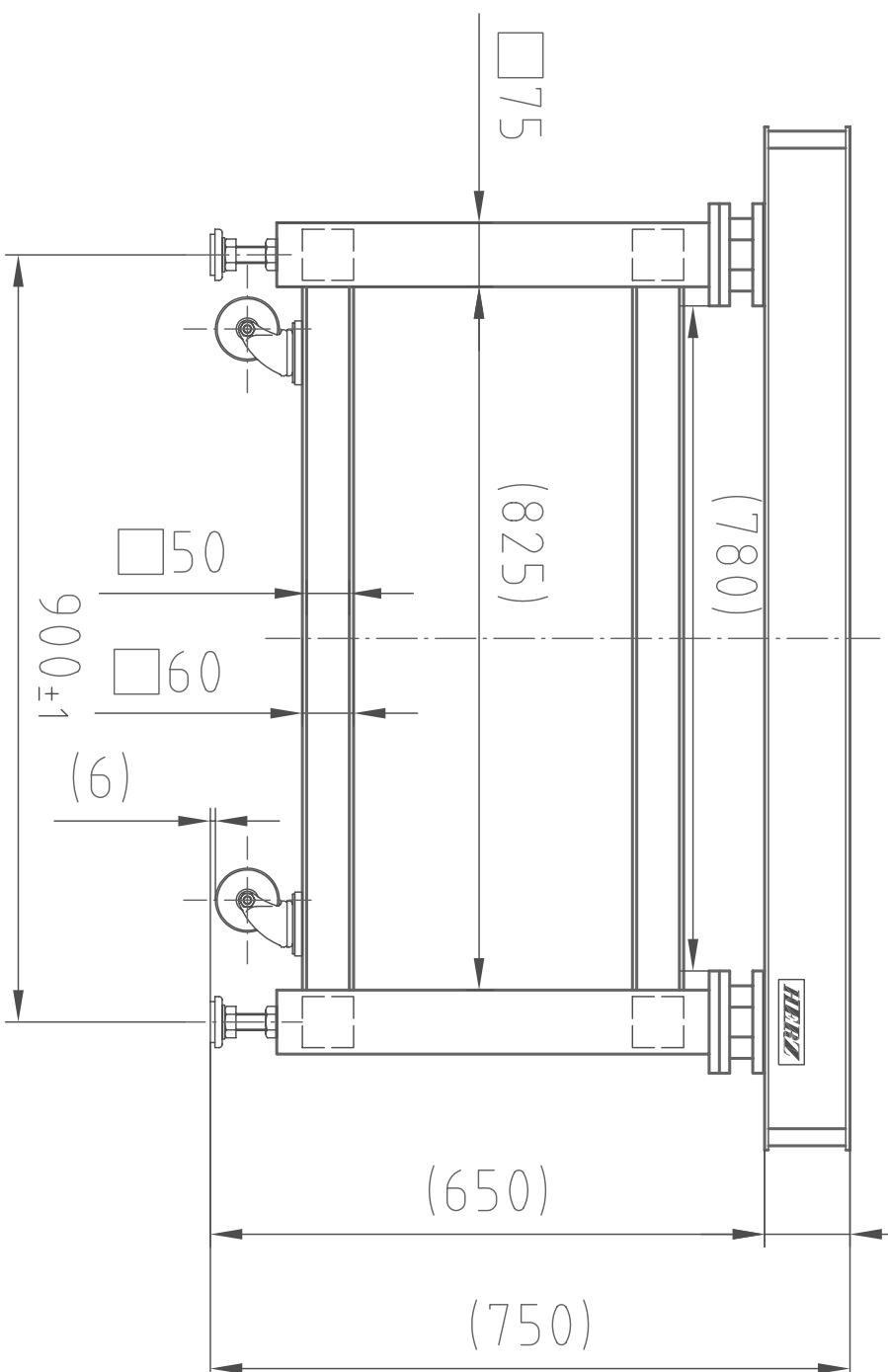
(正面図)
