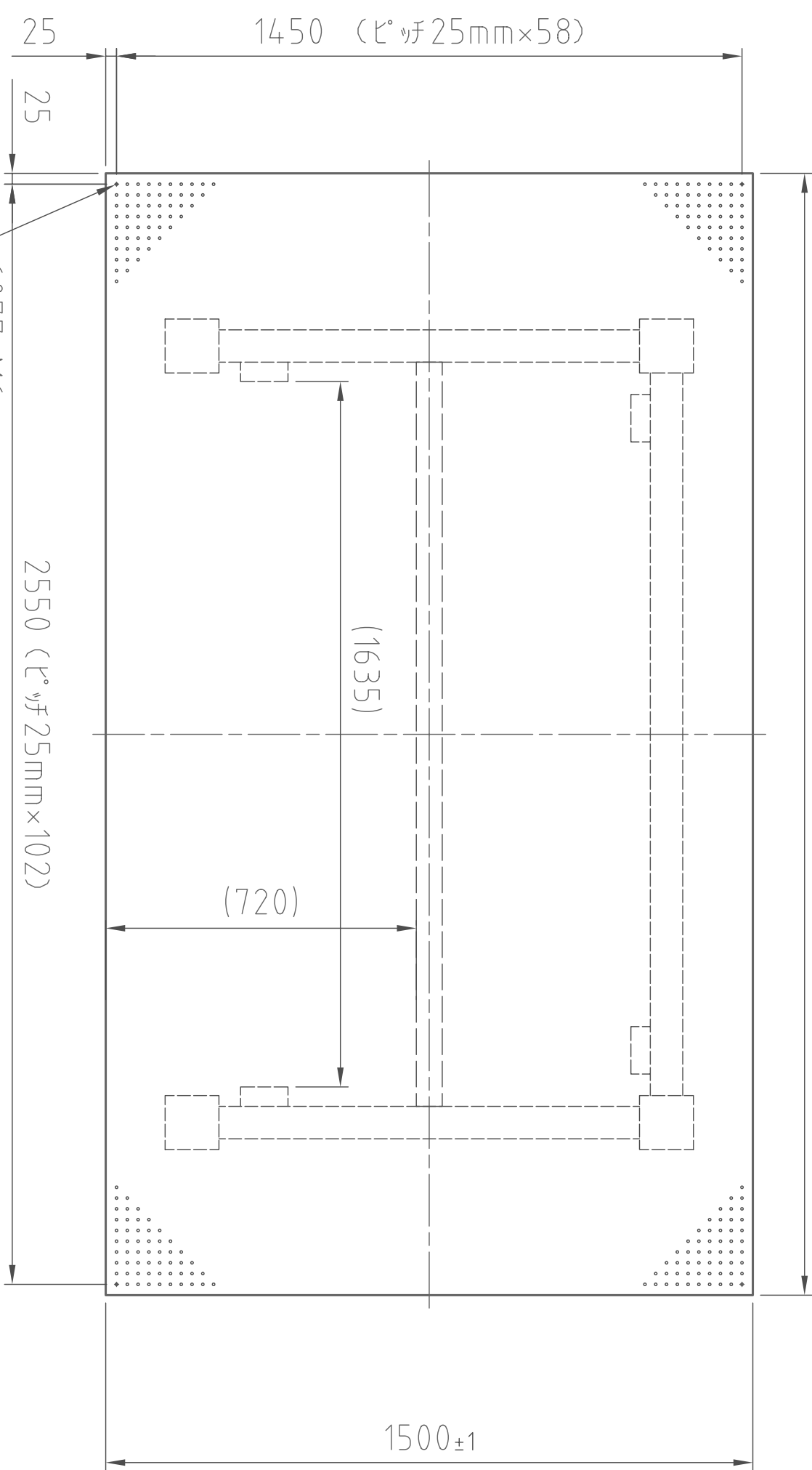
(平面図)
