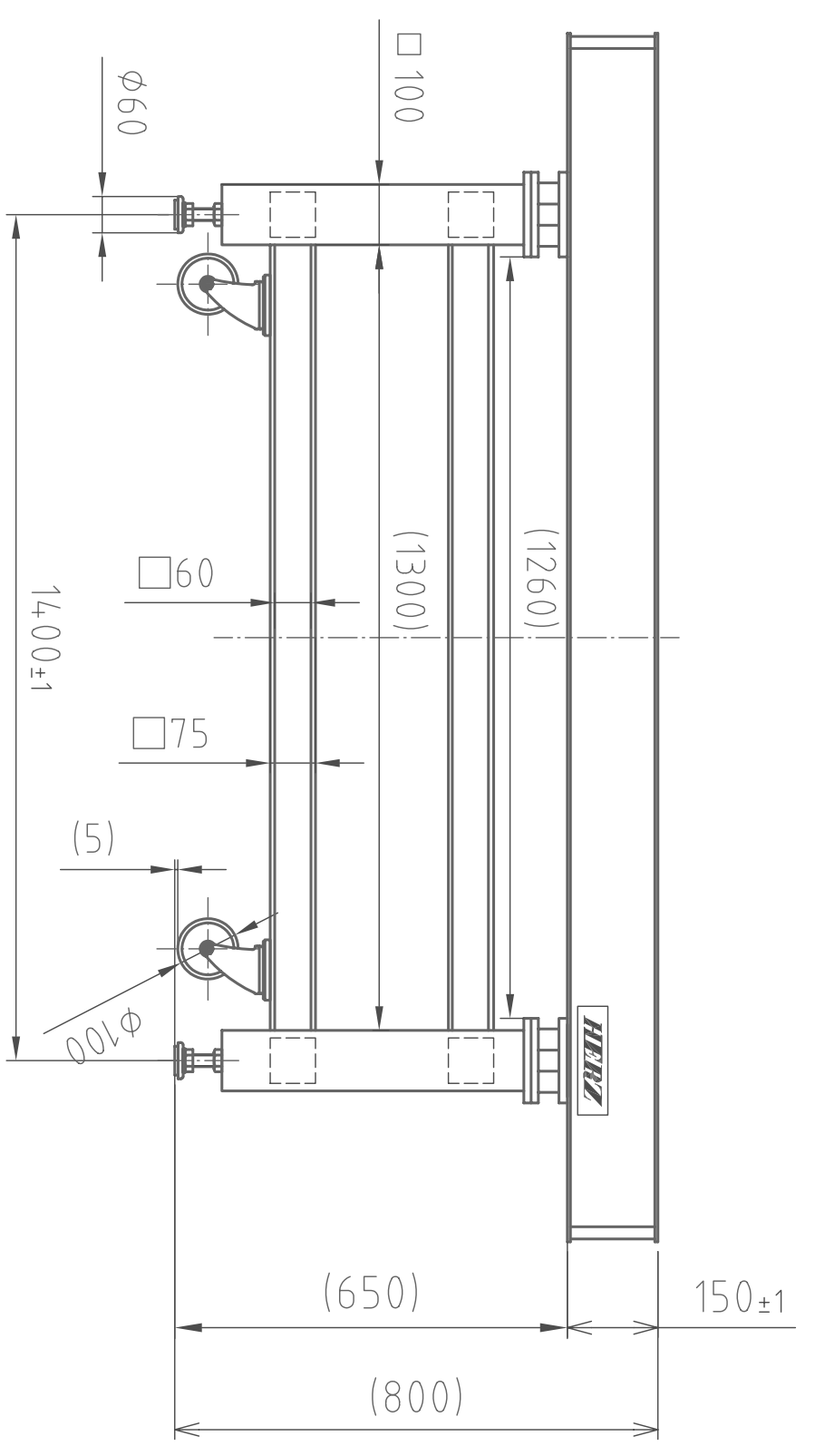
(正面図)
