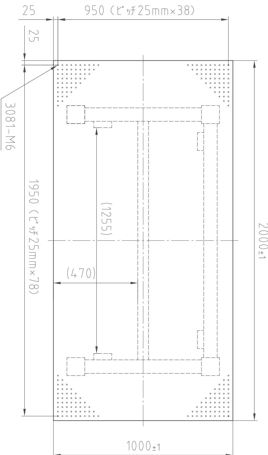
(平面図)
