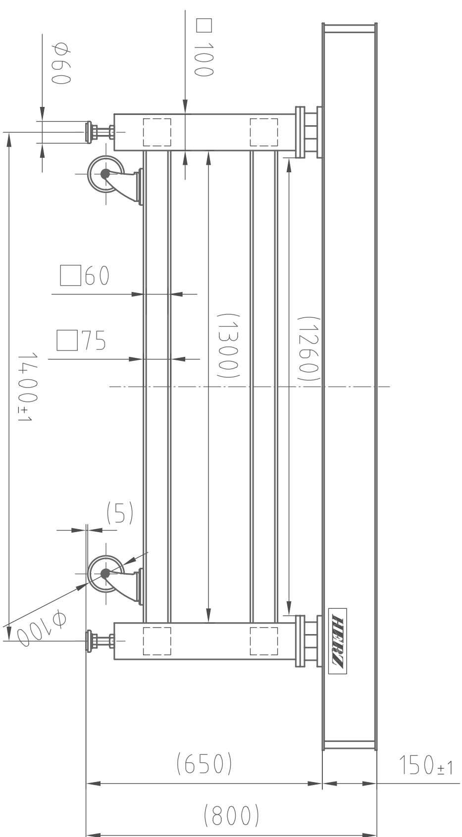
(正面図)
