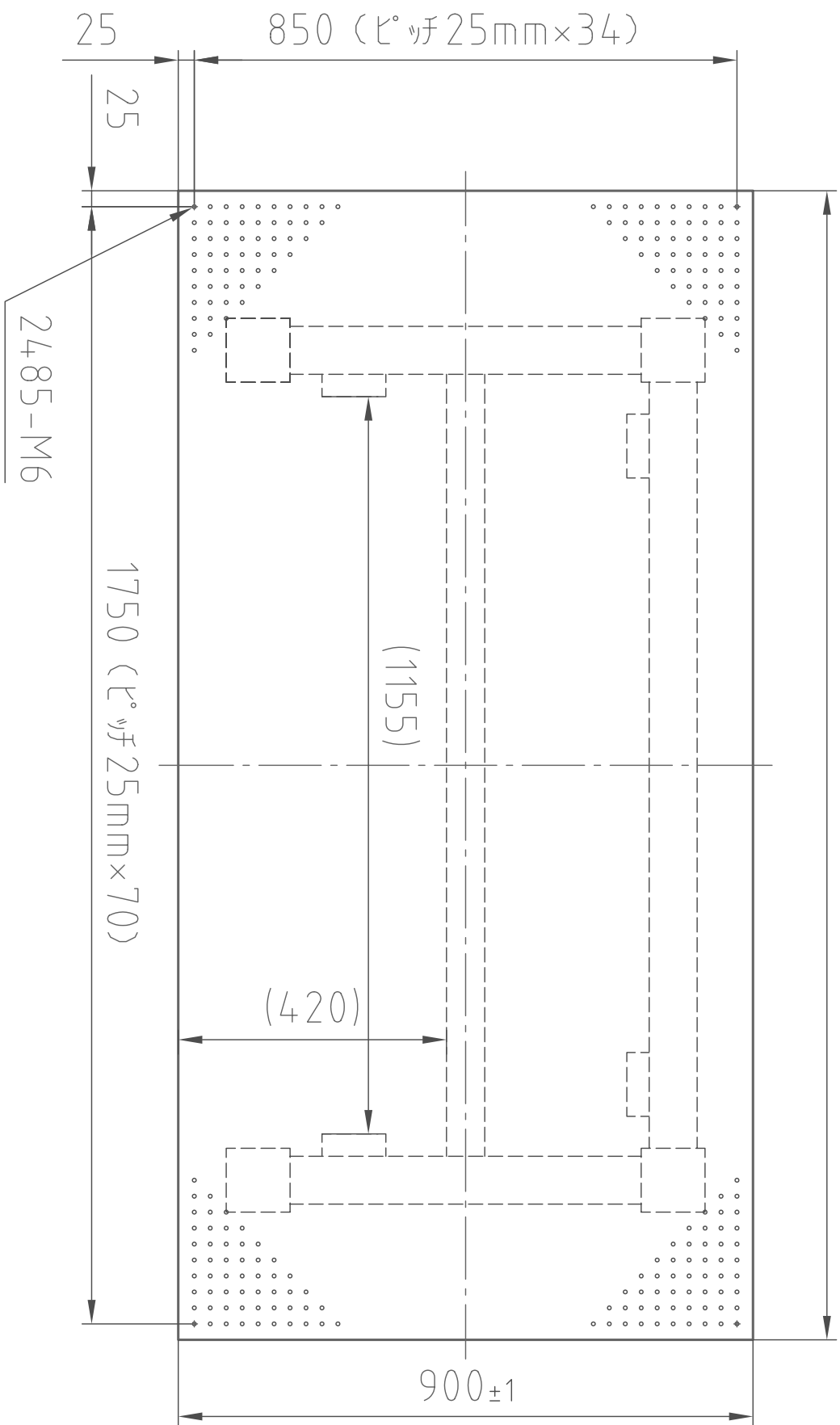
(平面図)
