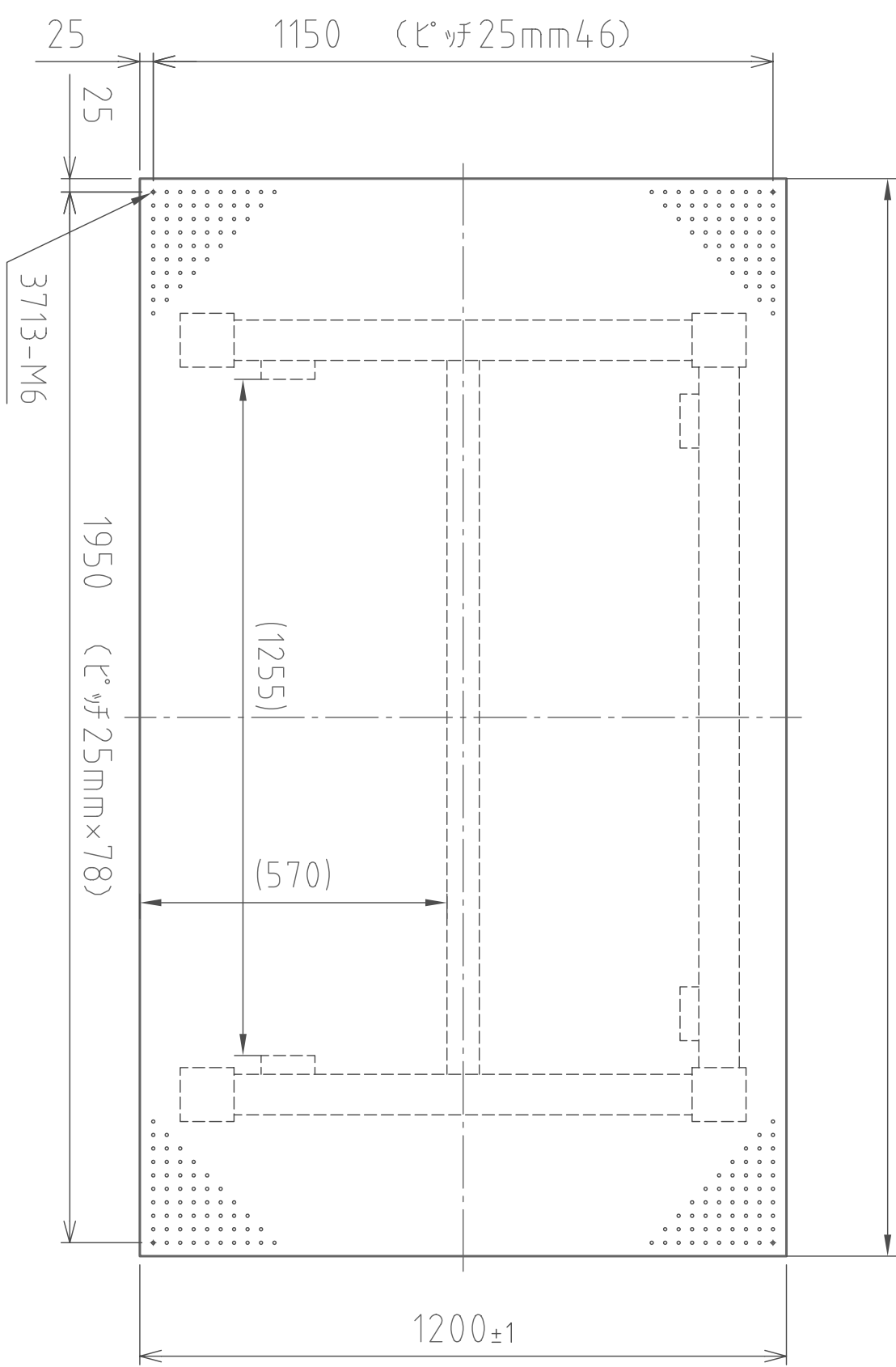
(平面図)
