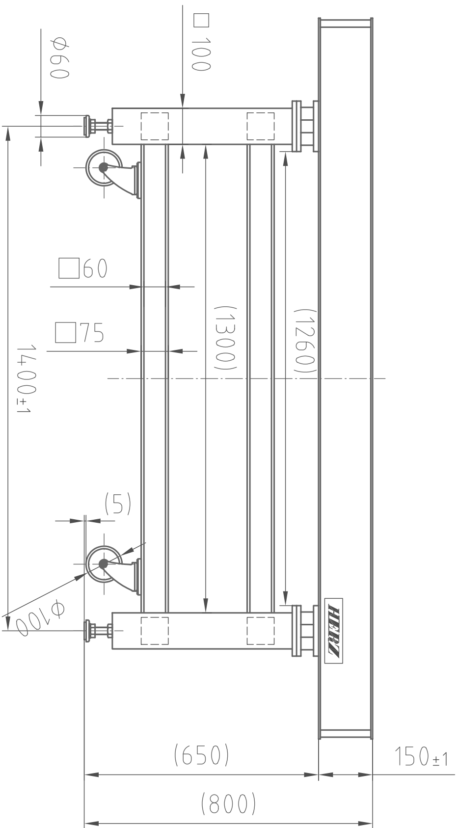
(正面図)
