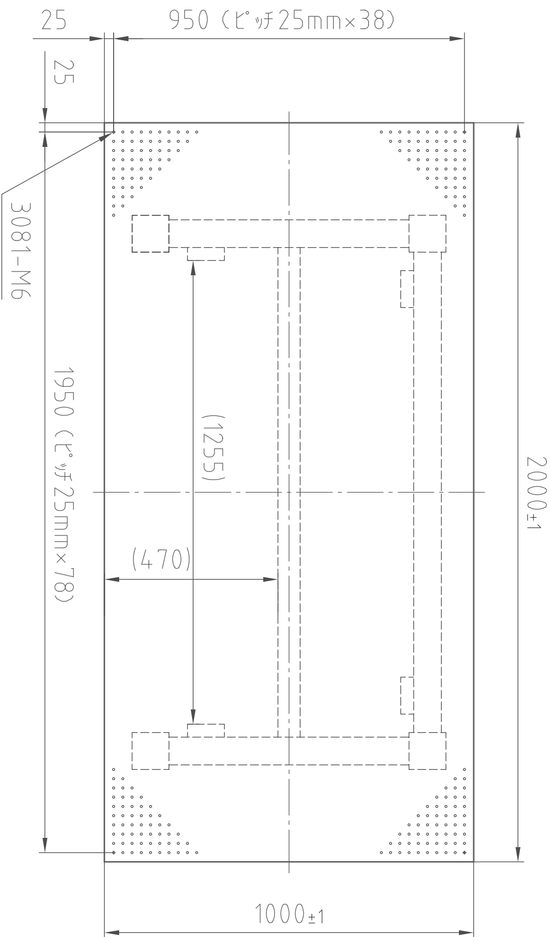
(平面図)
