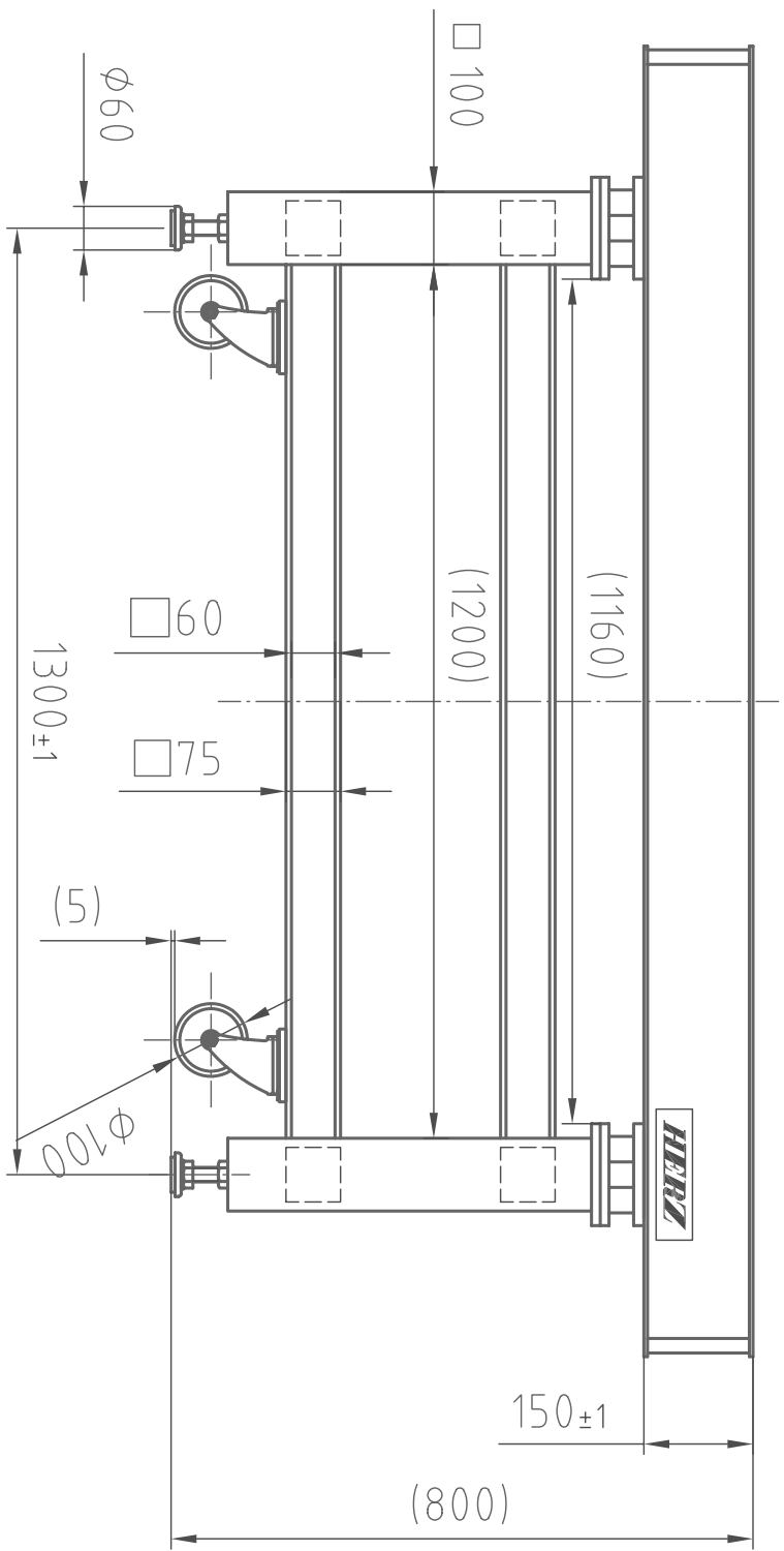
(正面図)
