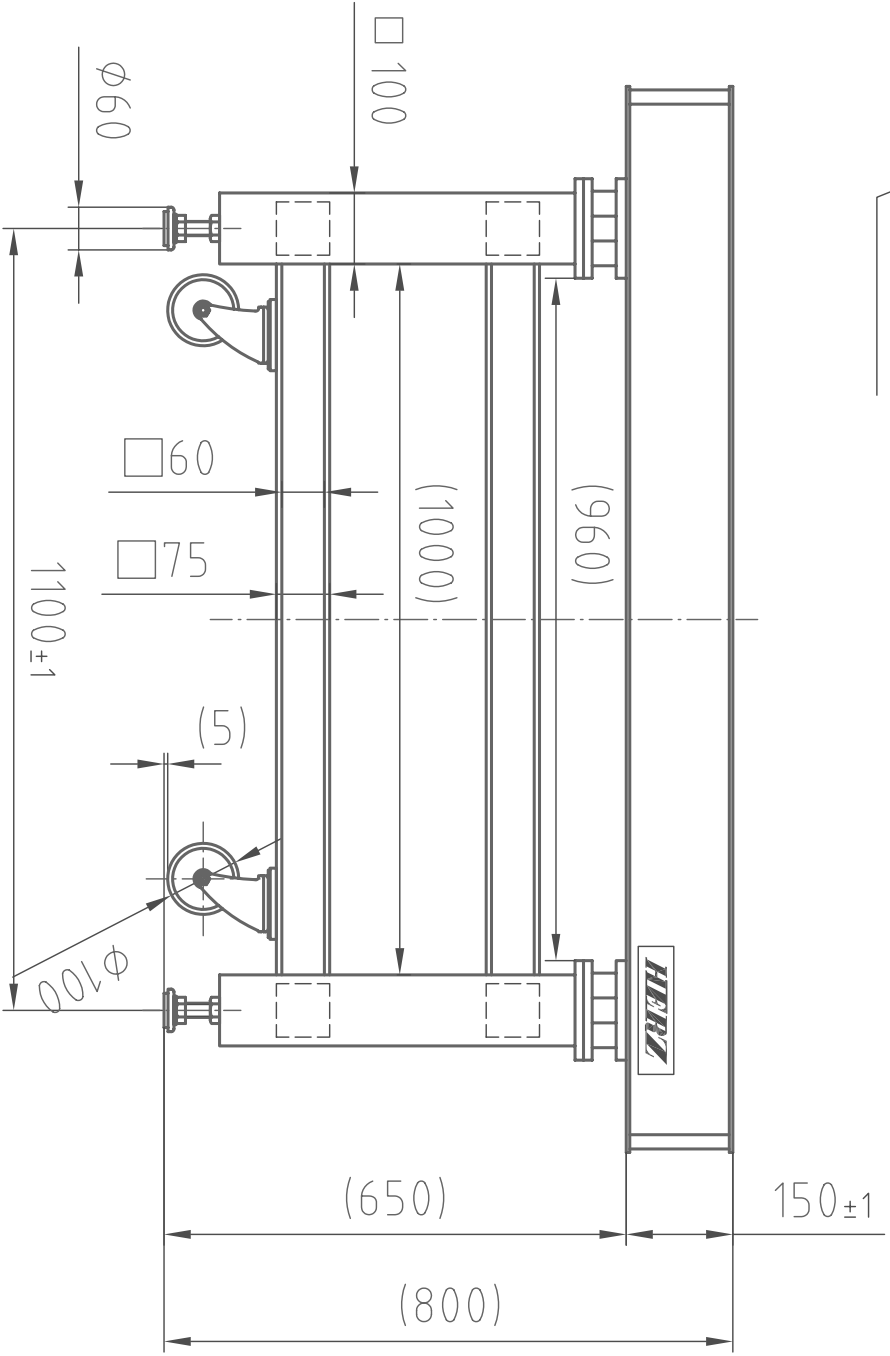
(正面図)
