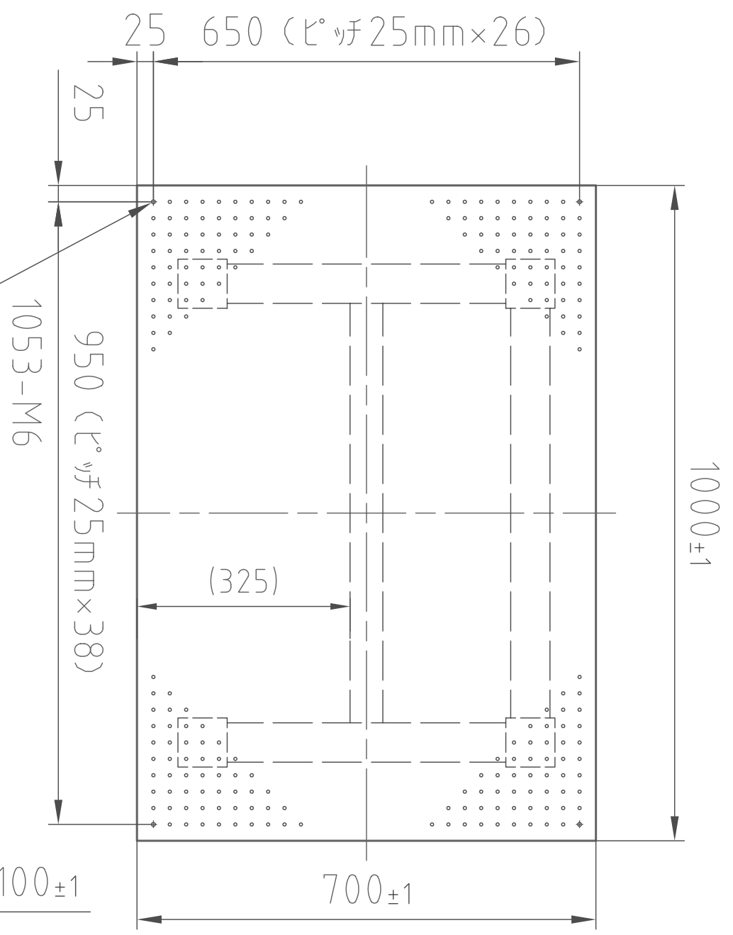
(平面図)
