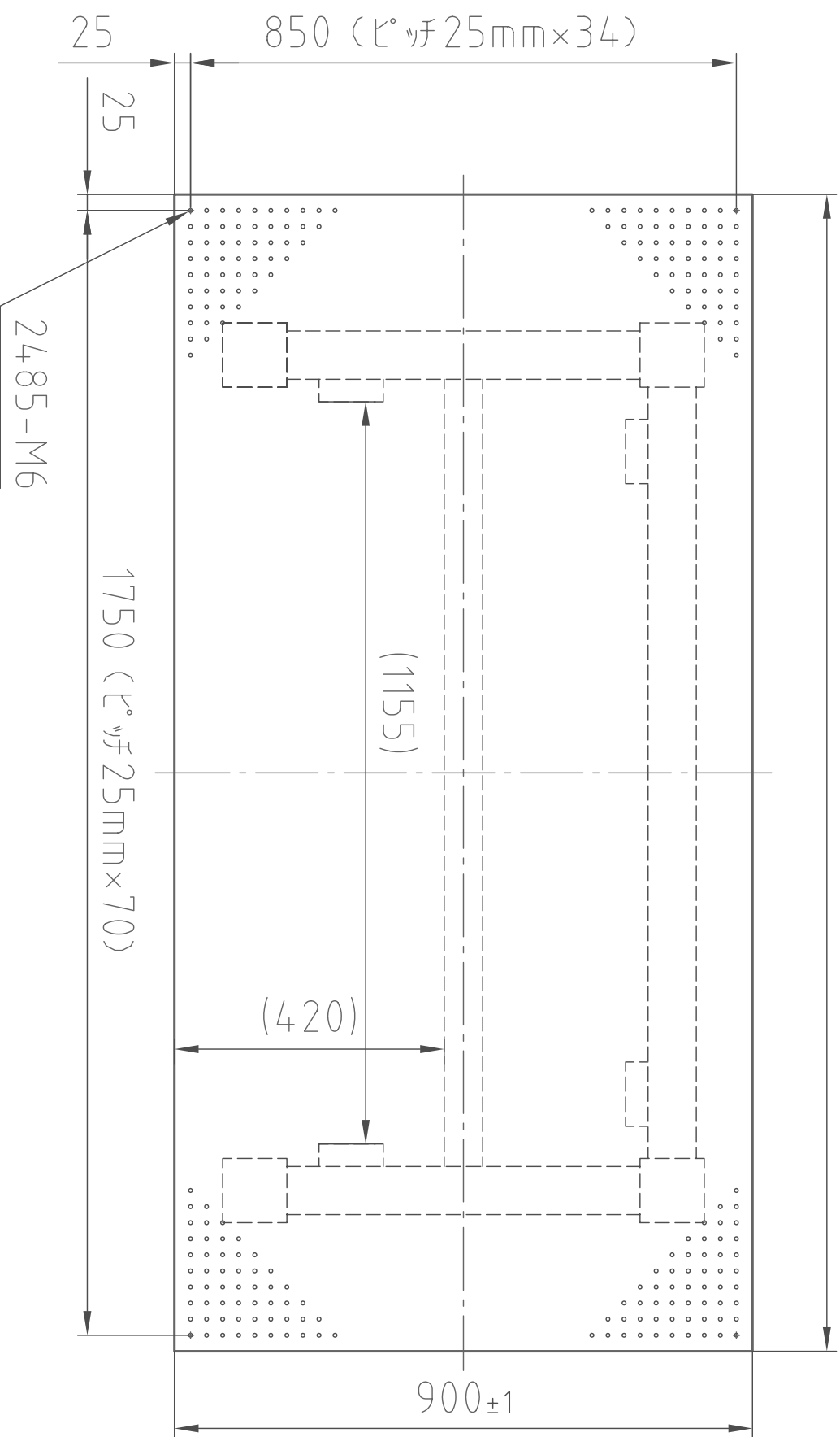
(平面図)
