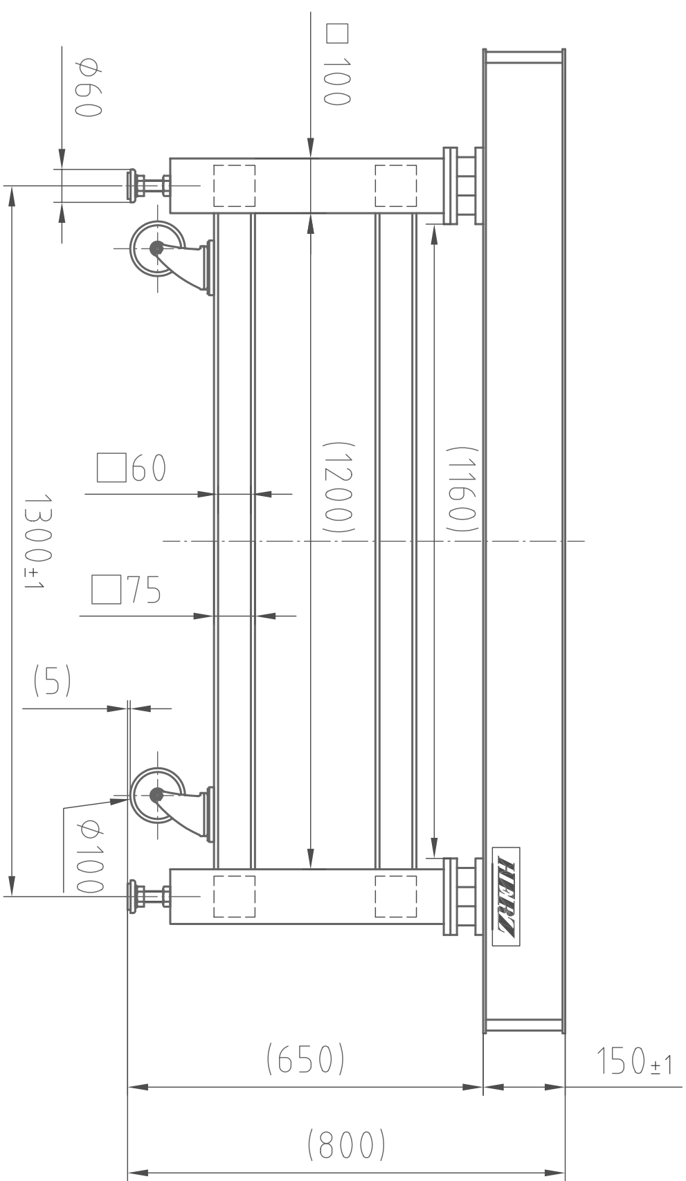
(正面図)
