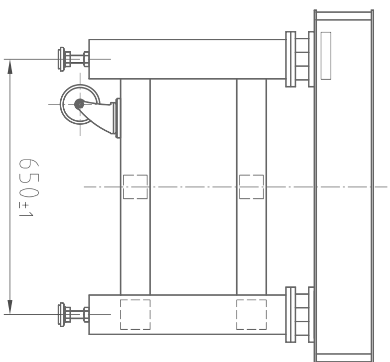
(右側面図)
