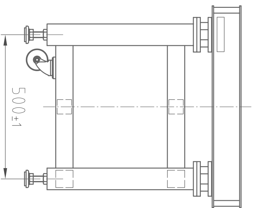
(右側面図)
