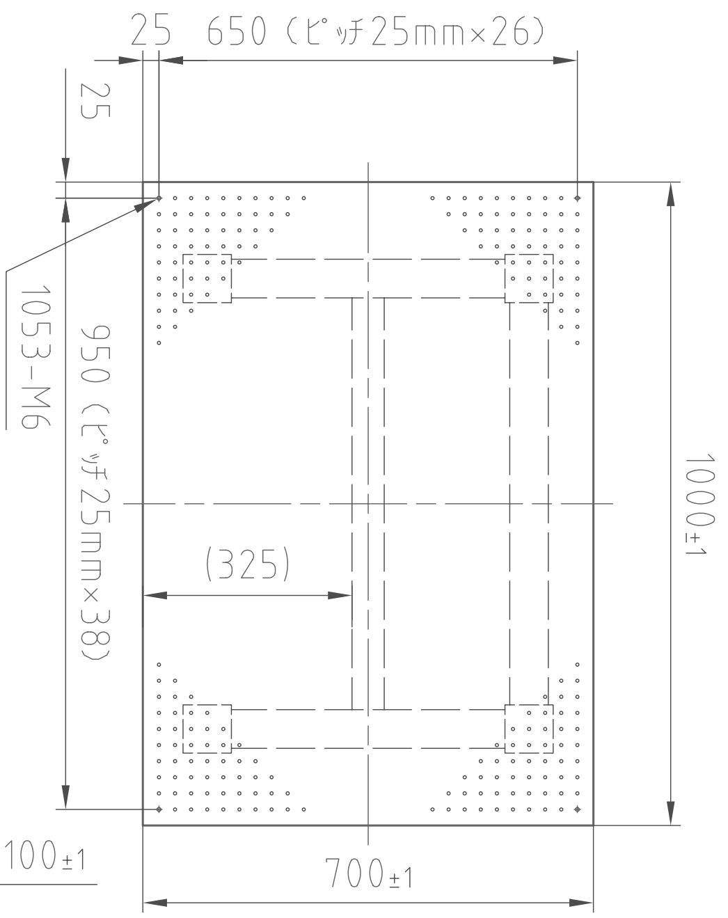
(平面図)
