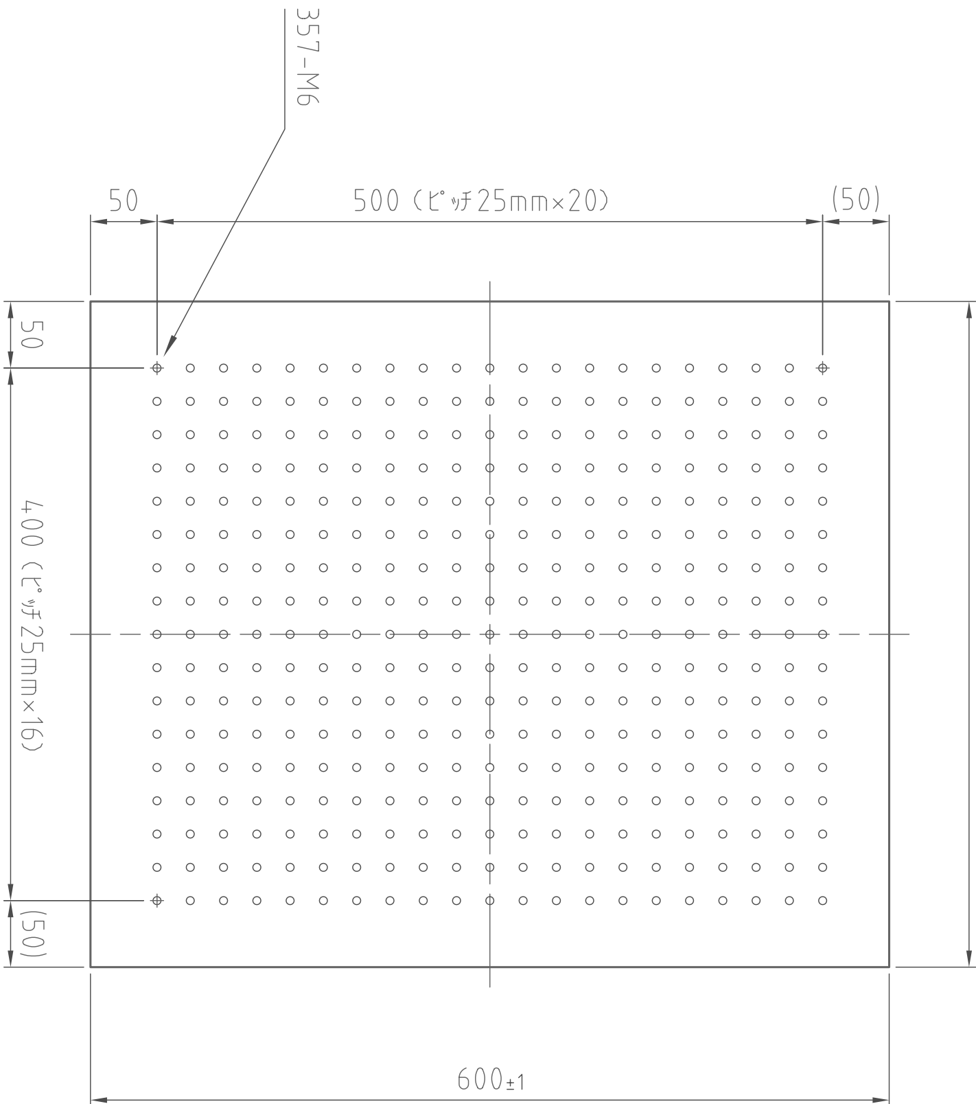
(平面図)
