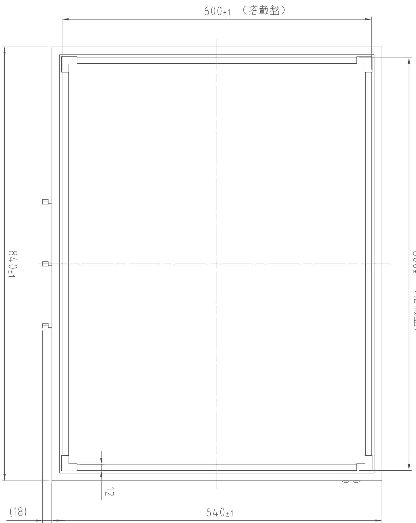
(平面図)
