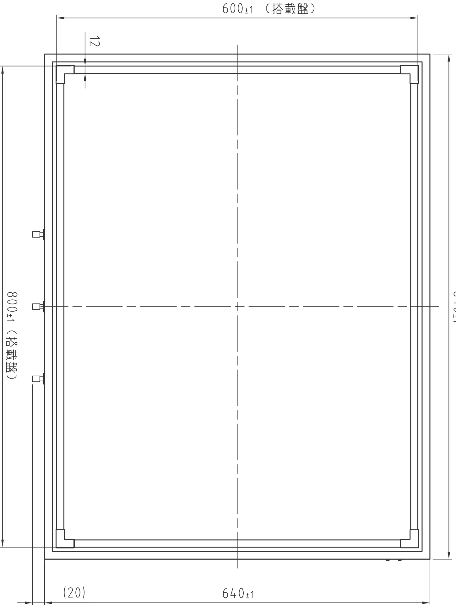
(平面図)
