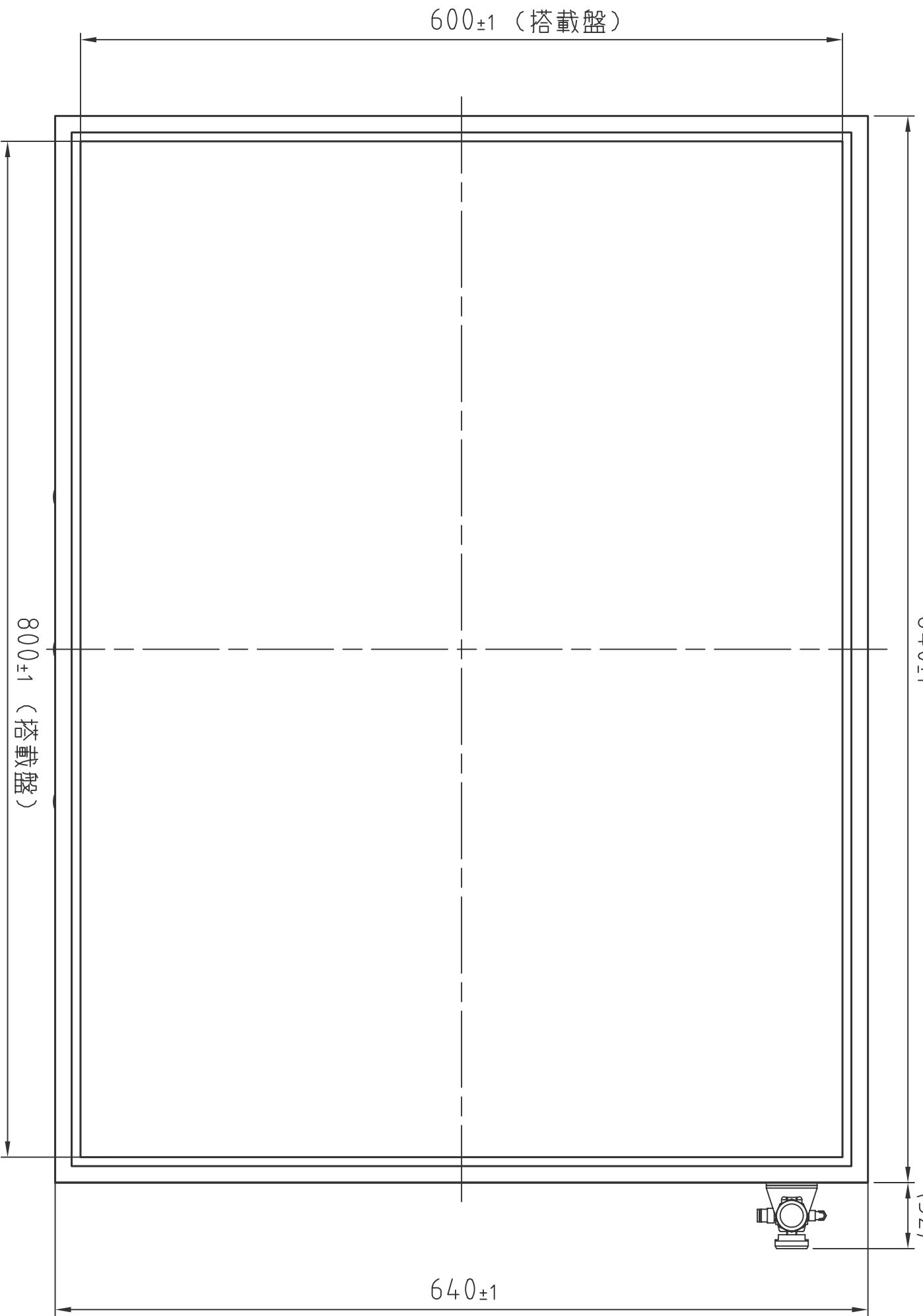
(平面図)
