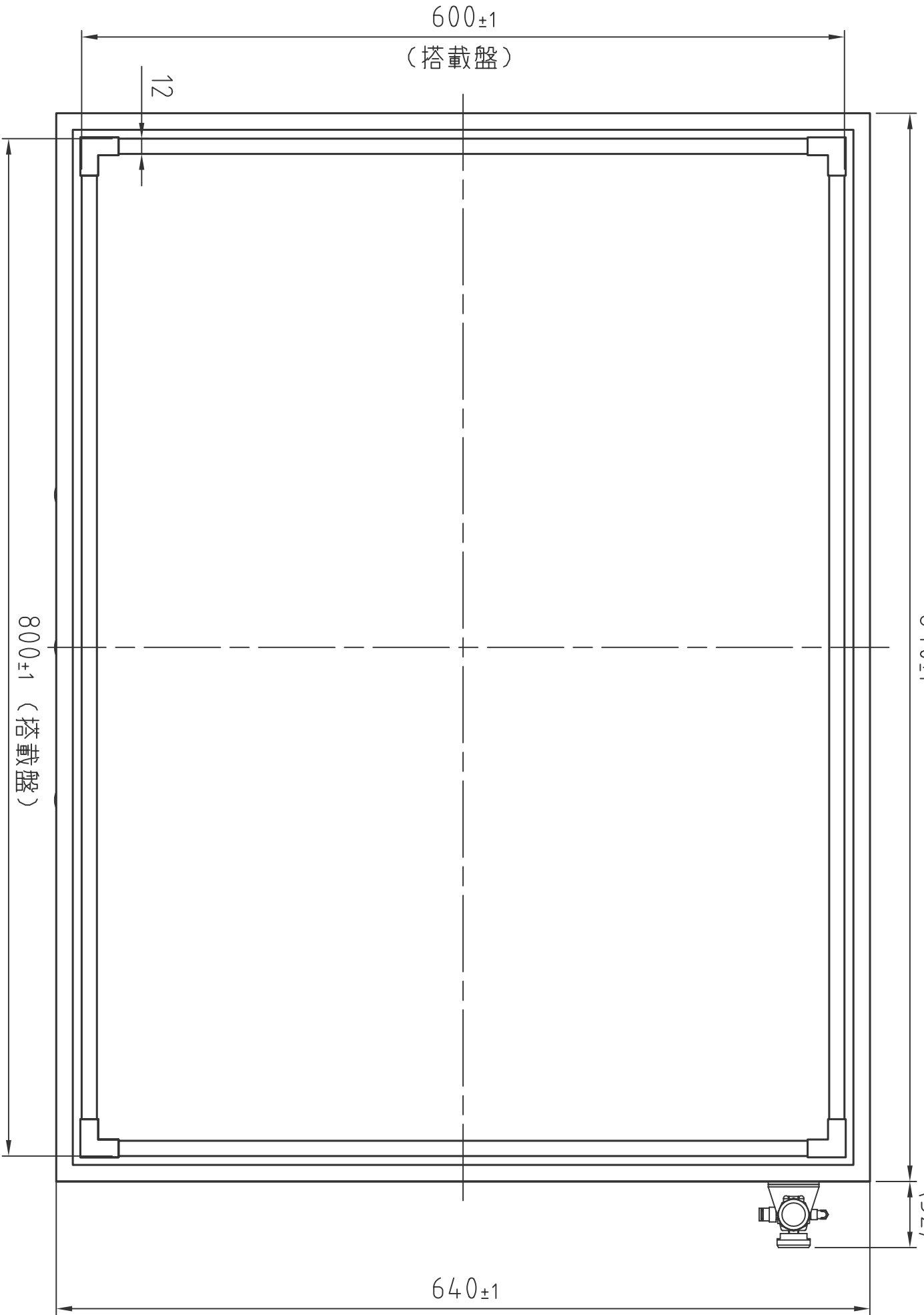
(平面図)
